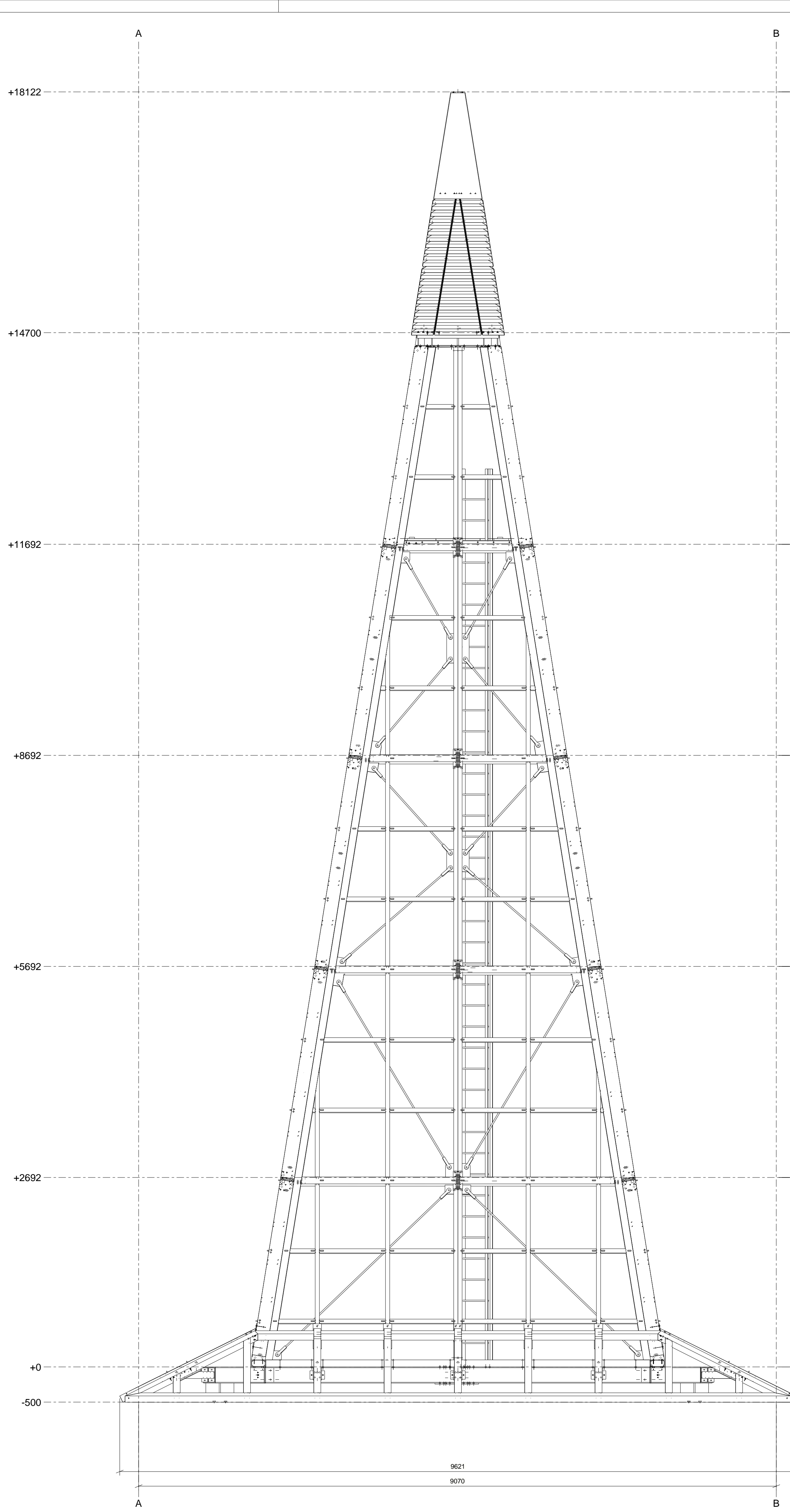
Aanzicht as 1 1:35
