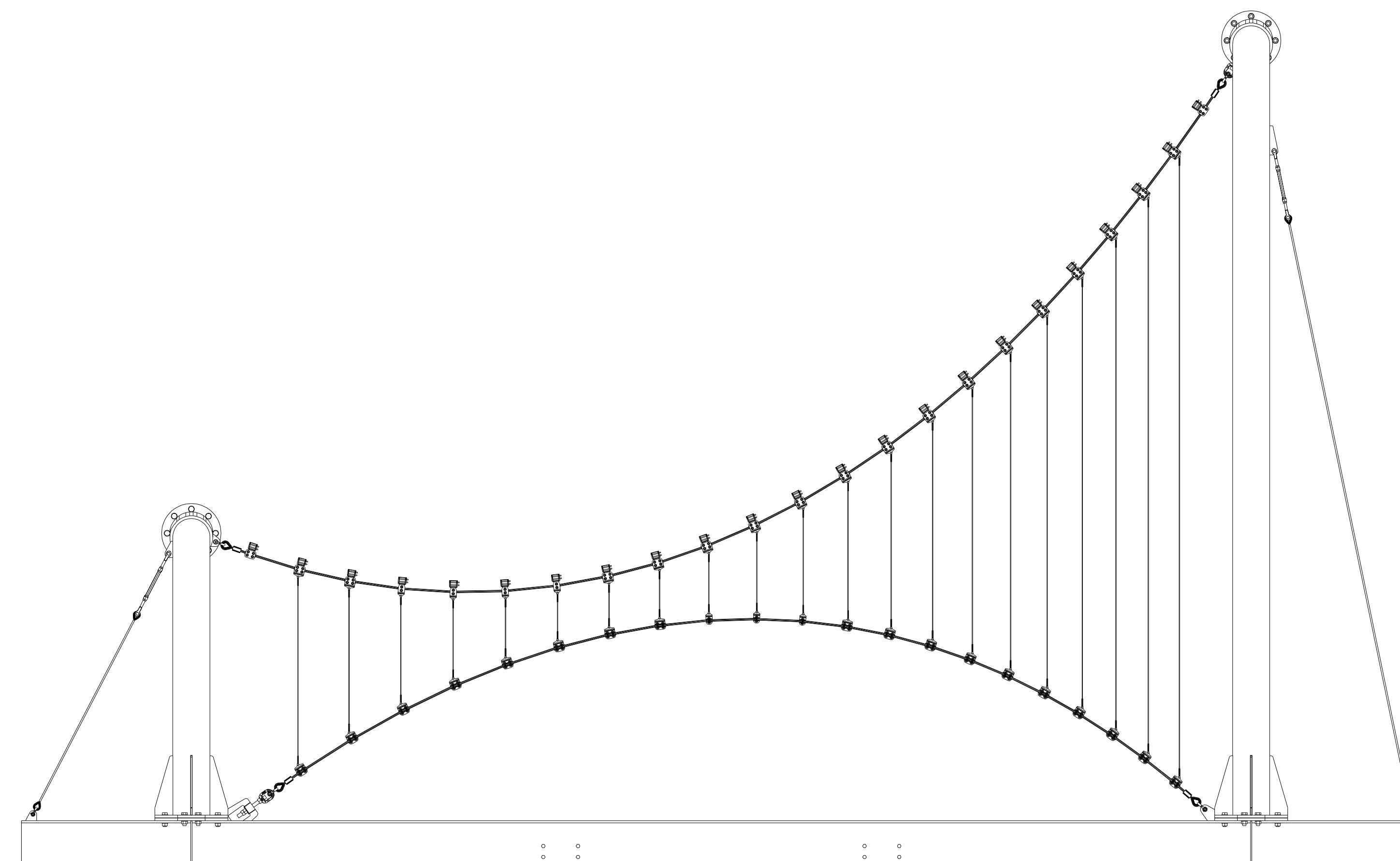
Zij aanzicht
