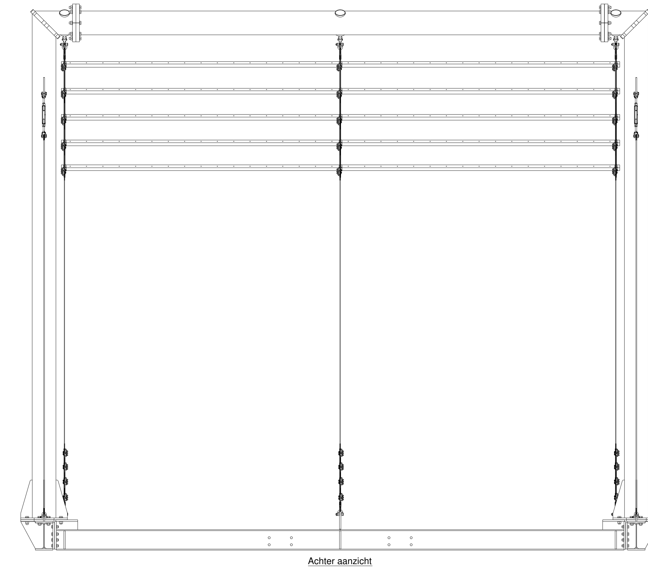
Achter aanzicht
