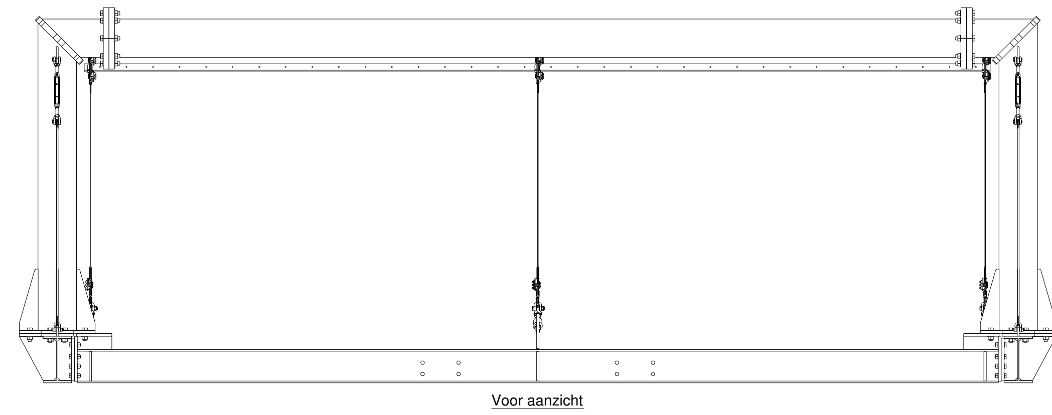
Voor aanzicht
