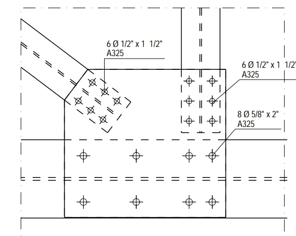
DETALLE 1 1:10
