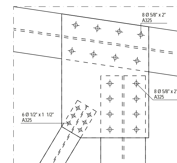
DETALLE 4 1:10
