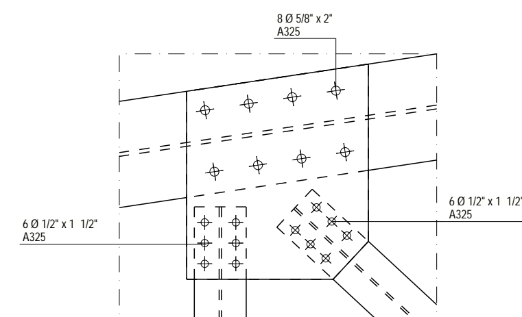
DETALLE 2 1:10
