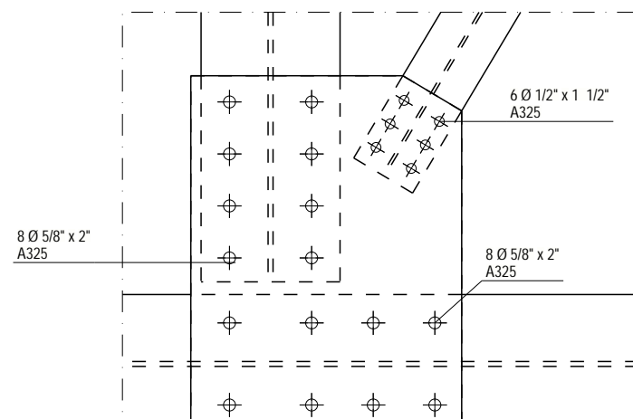
DETALLE 3 1:10
