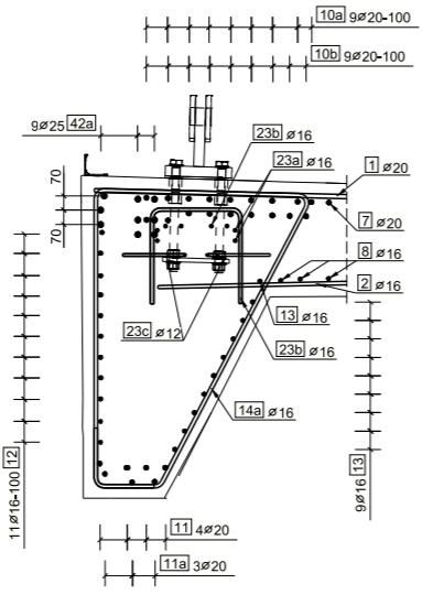
Section D - D HDPE GUIDE 1:20
