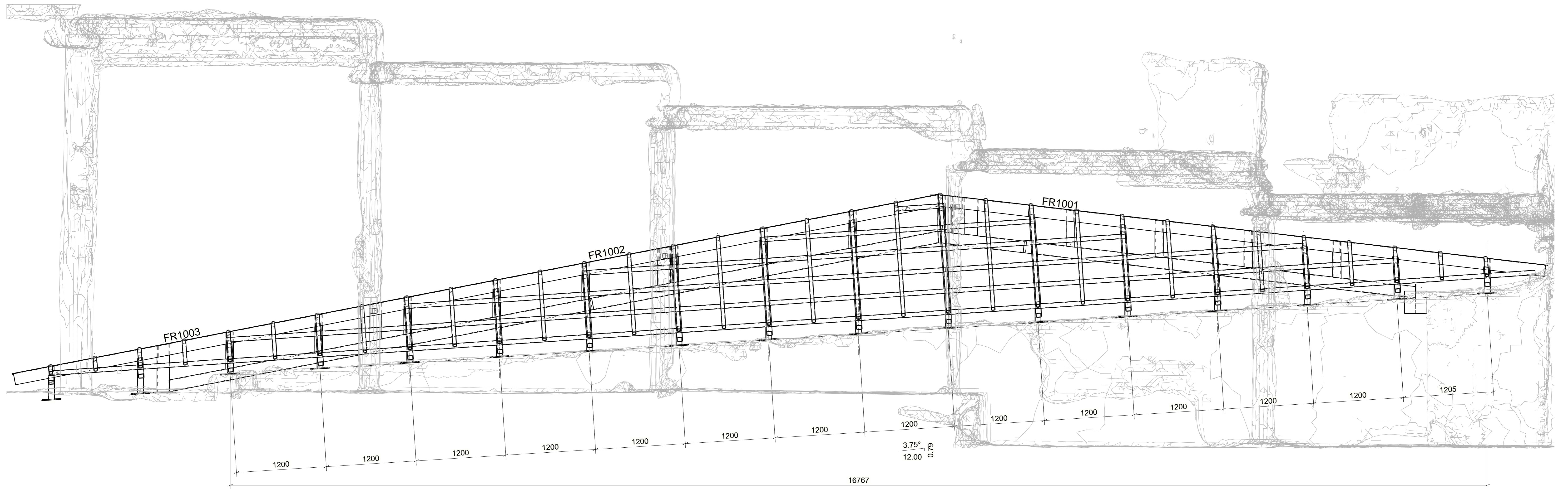
ELEVATION
