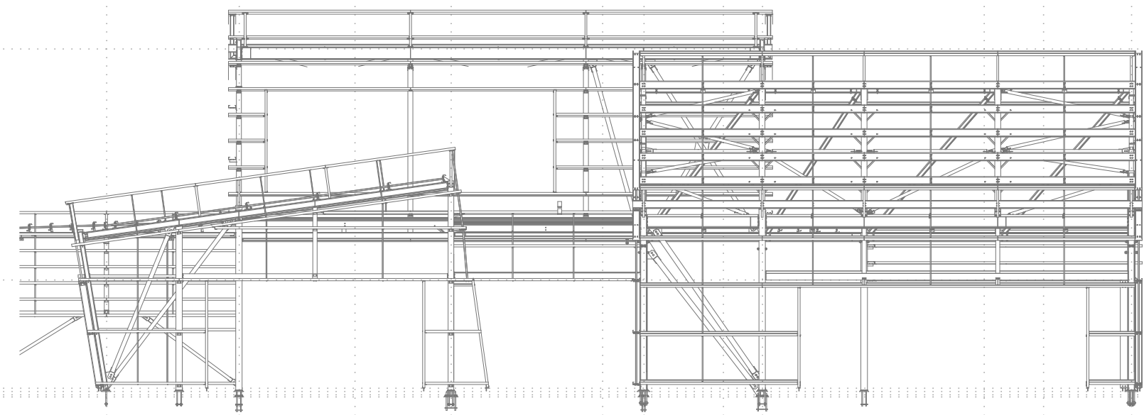
ALÇADO SUDESTE
