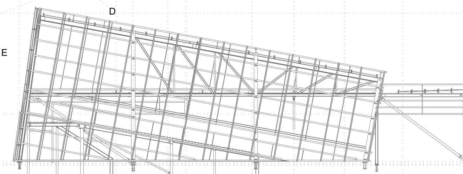
ALÇADO NOROESTE
