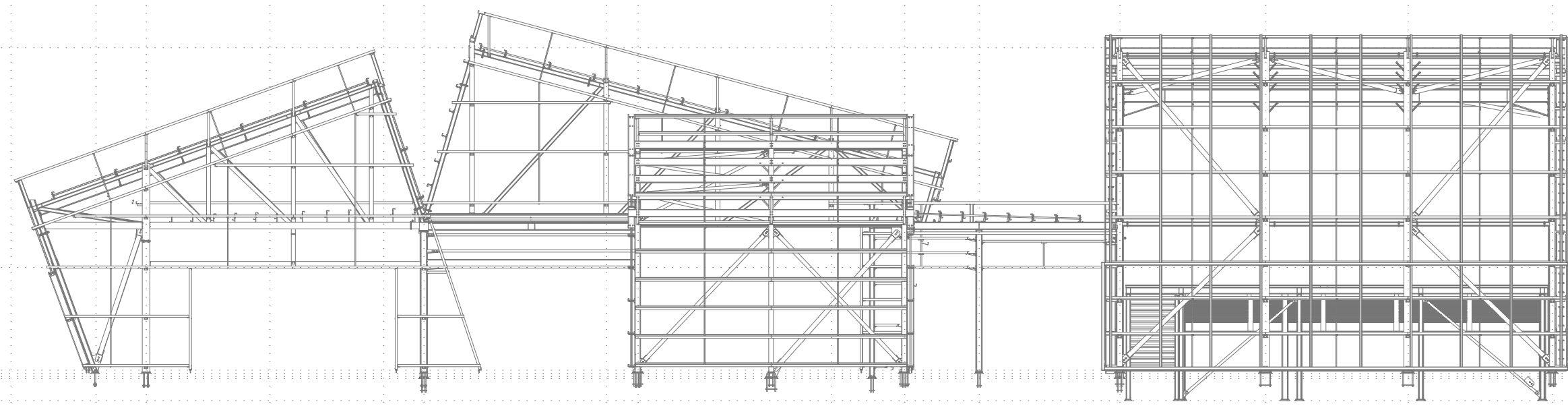
ALÇADO NORDESTE
