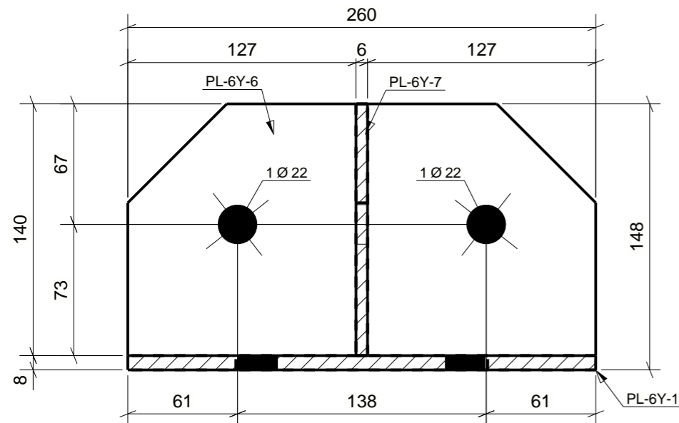
Seccion A - A Escala: 1:3
