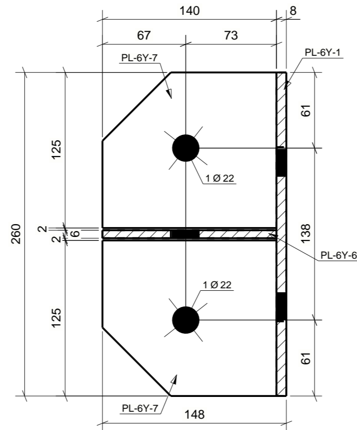
Seccion B - B Escala: 1:3
