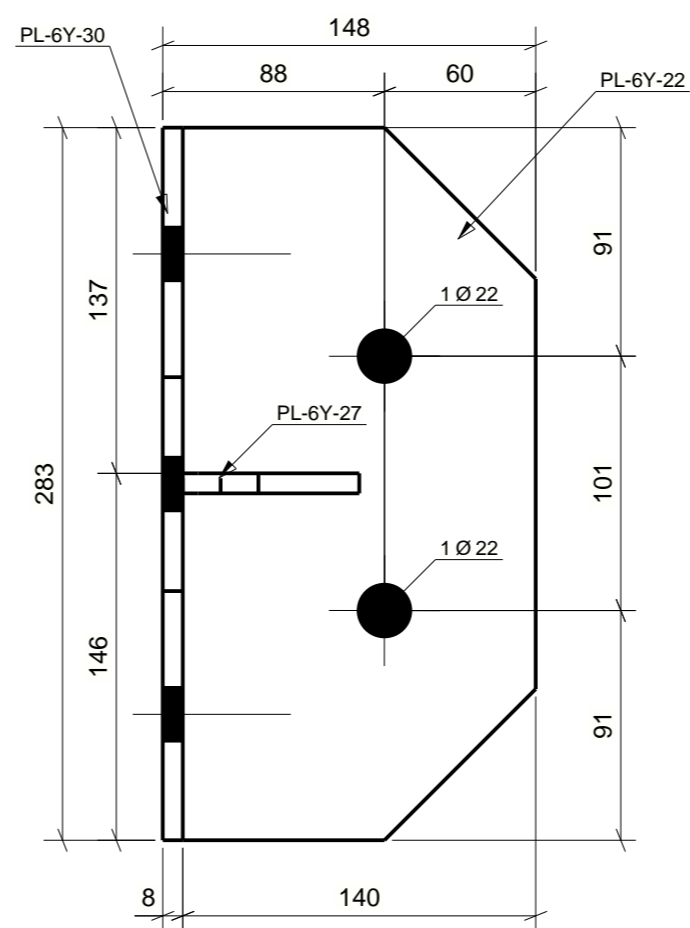
Seccion A - A Escala: 1:3
