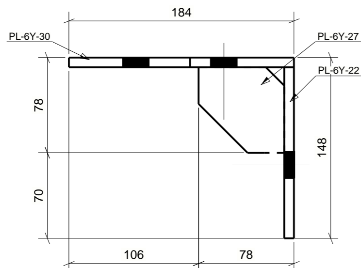
Seccion B - B Escala: 1:3
