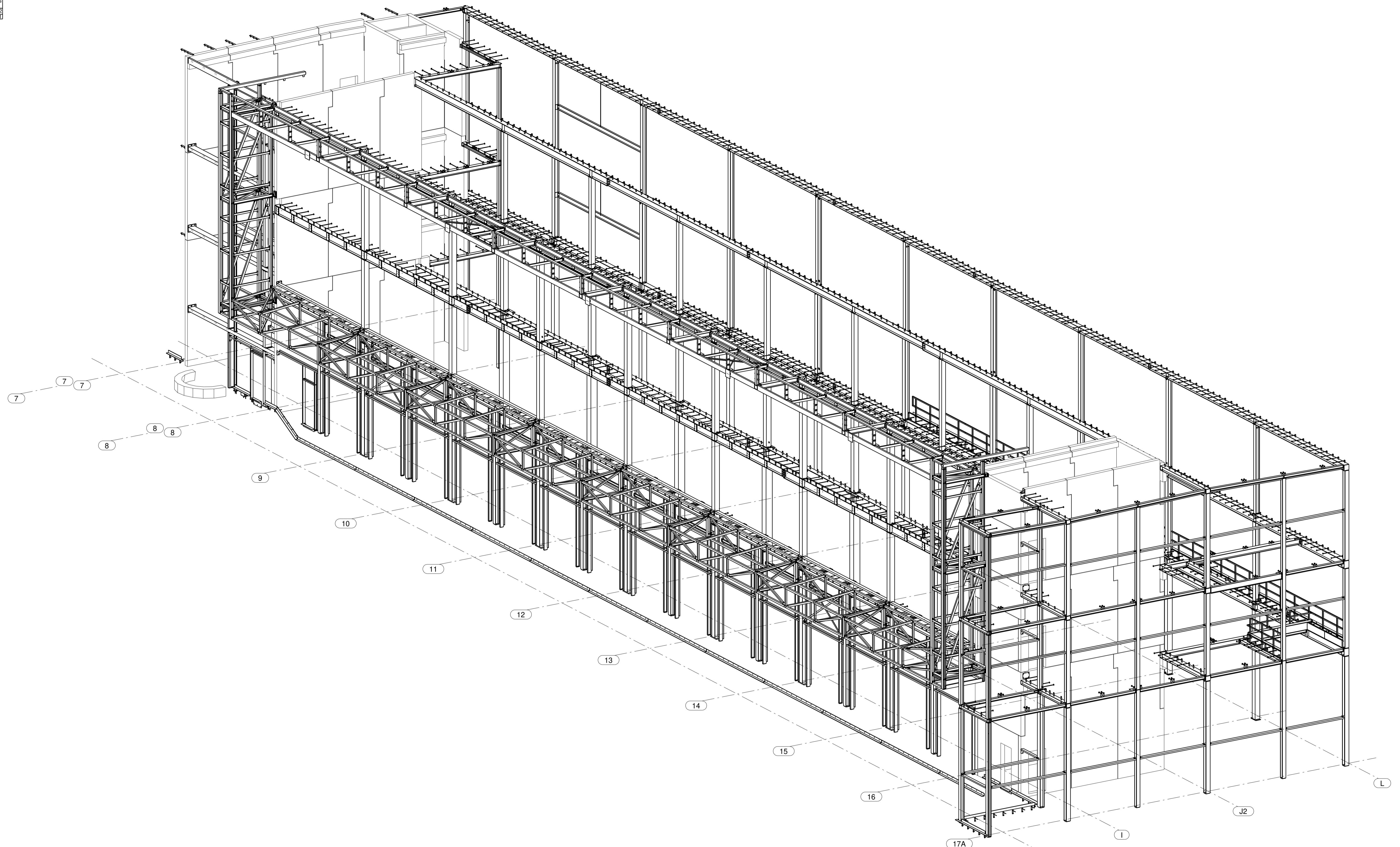
3D OVERZICHT 1:100
