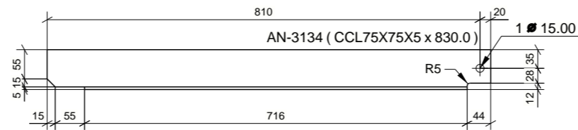
FRONT VIEW / VISTA FRONTAL SC. / ESC. 1:10
