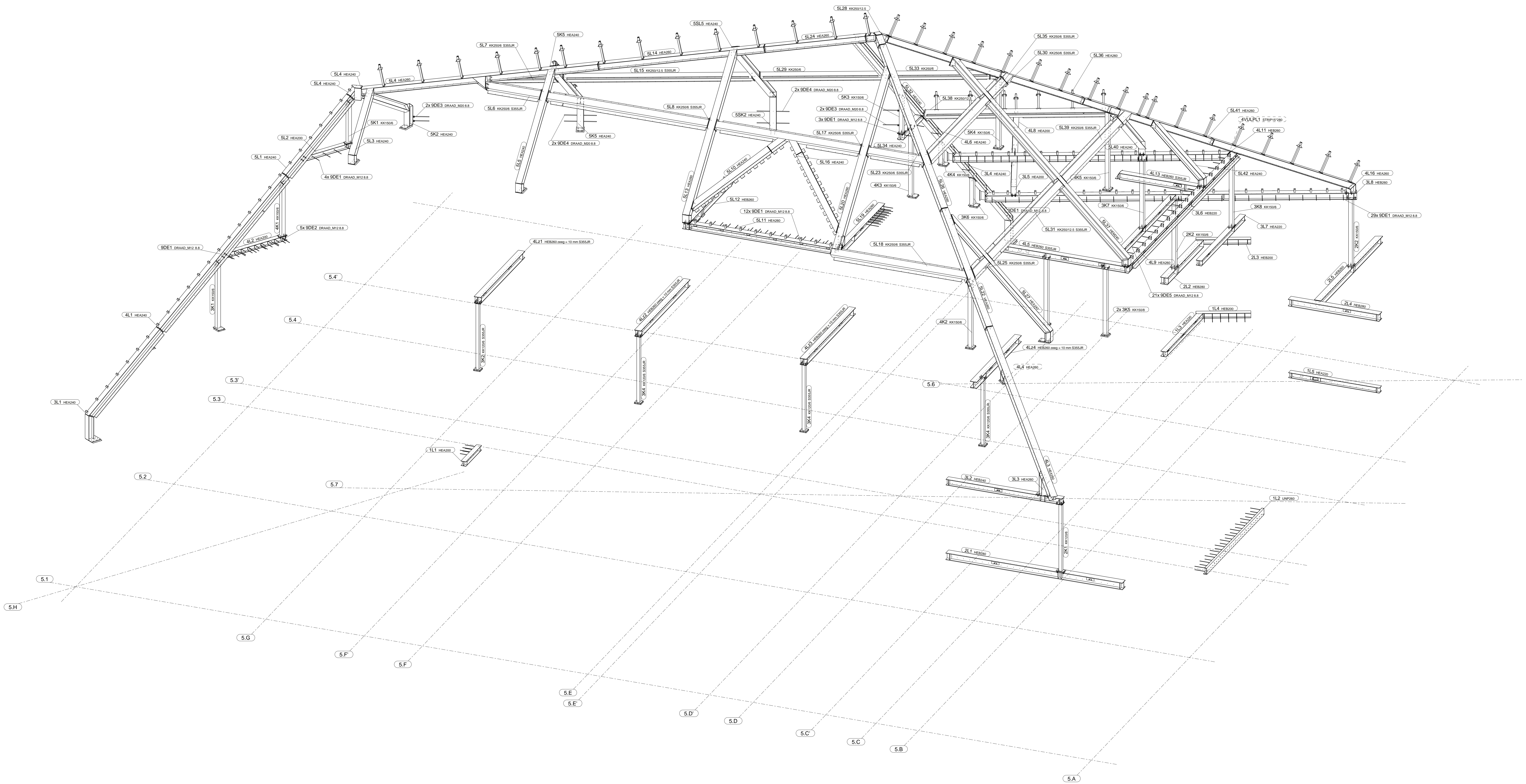
3D-AANZICHT 1:50
