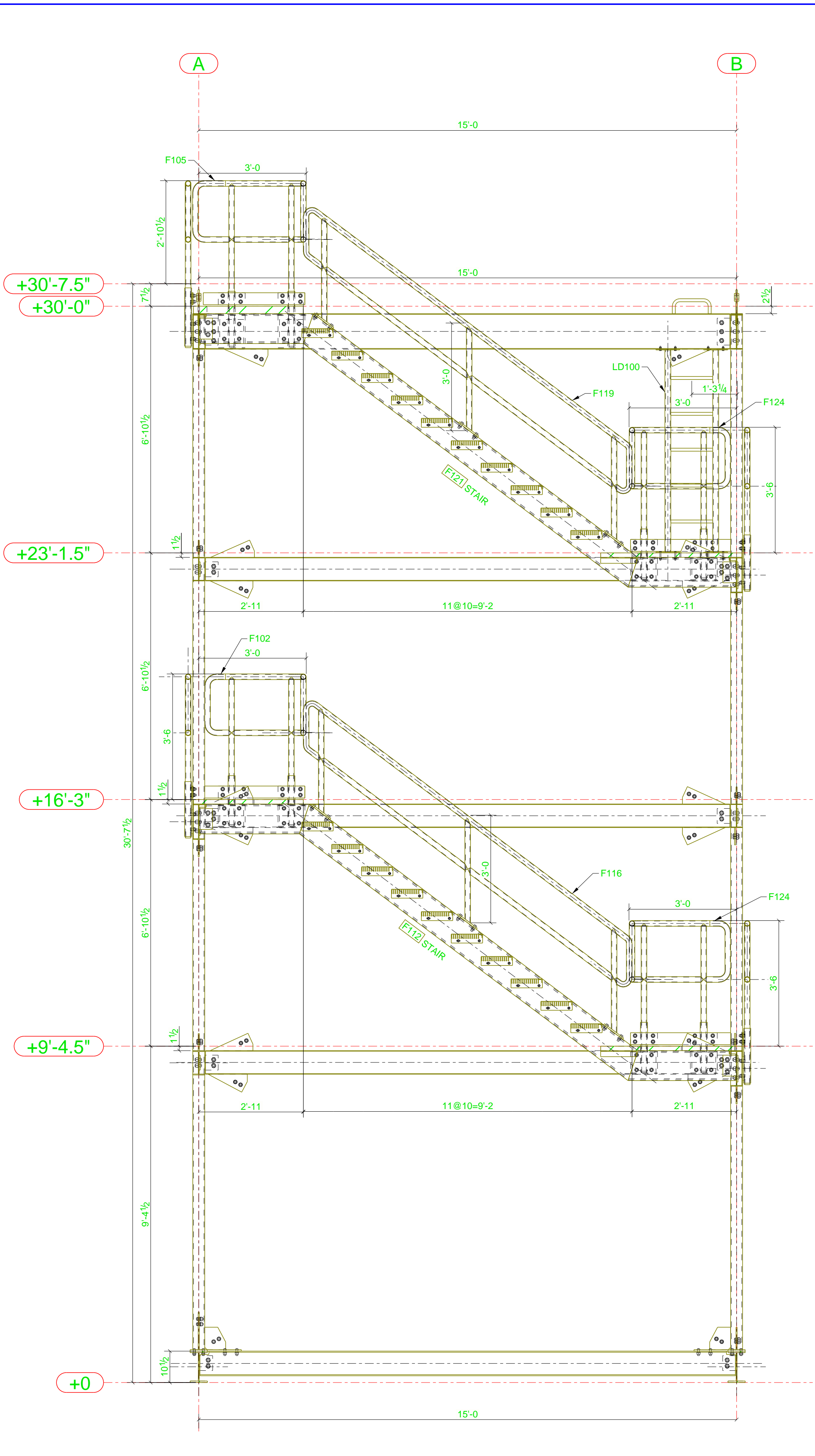
F ELEVATION F104 REF: E100
