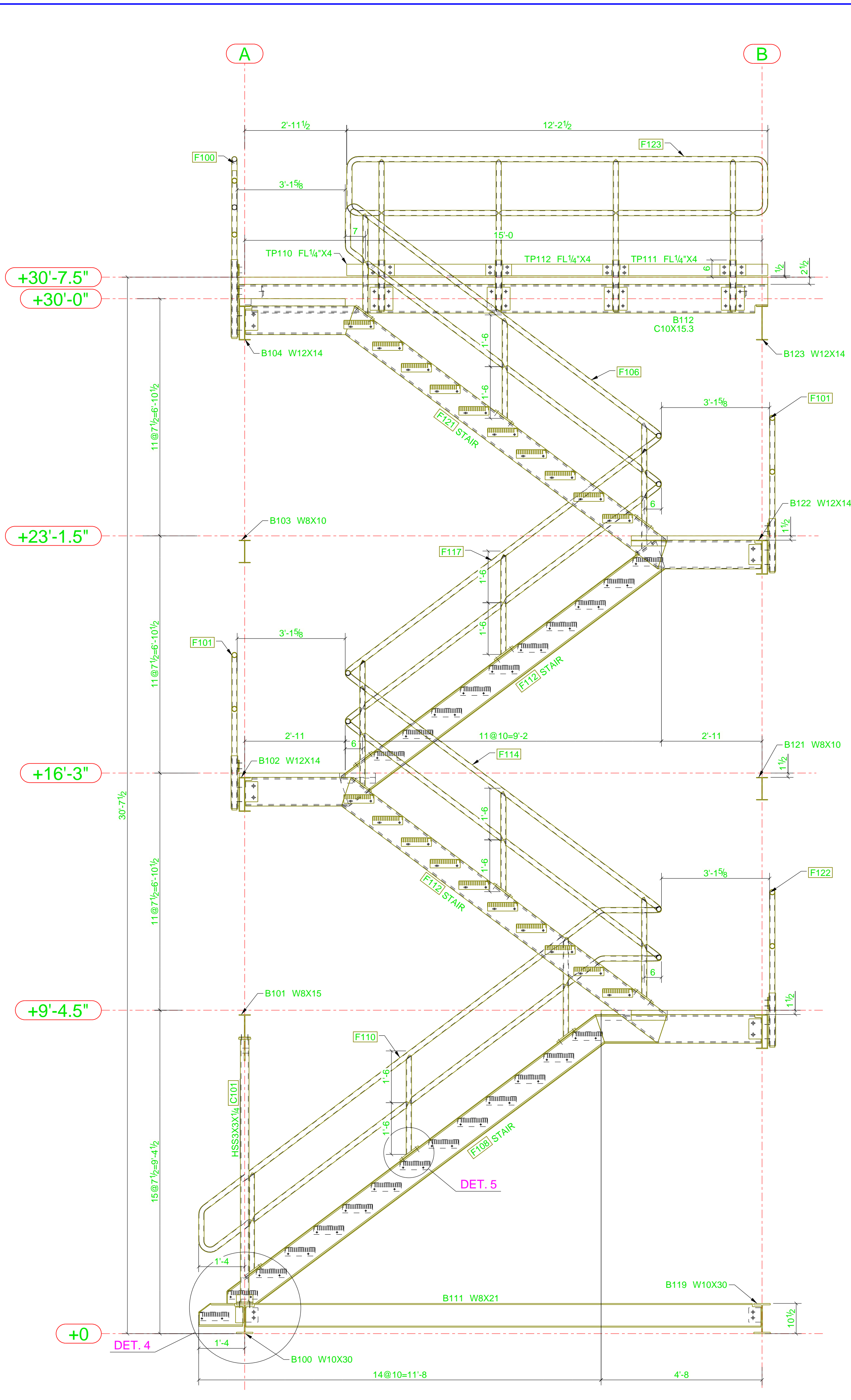
E ELEVATION E104 REF: E100
