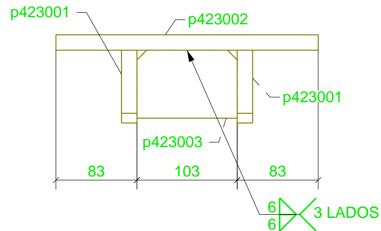
2 SECCION 2 - 2 ESC. 1:5
