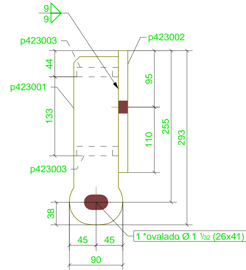
1 SECCION 1 - 1 ESC. 1:5
