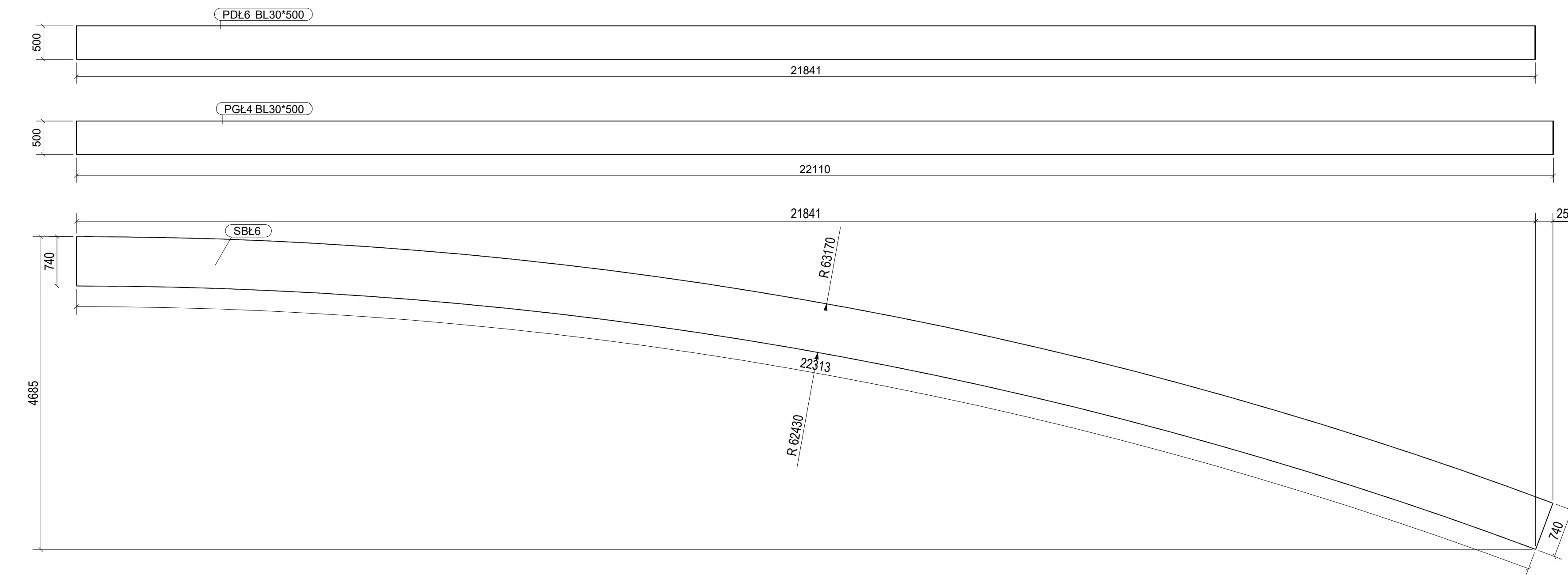
SEKCJA ŁUKU SP4 POJEDYNCZE BLACHY ŁUKU Skala 1:50
