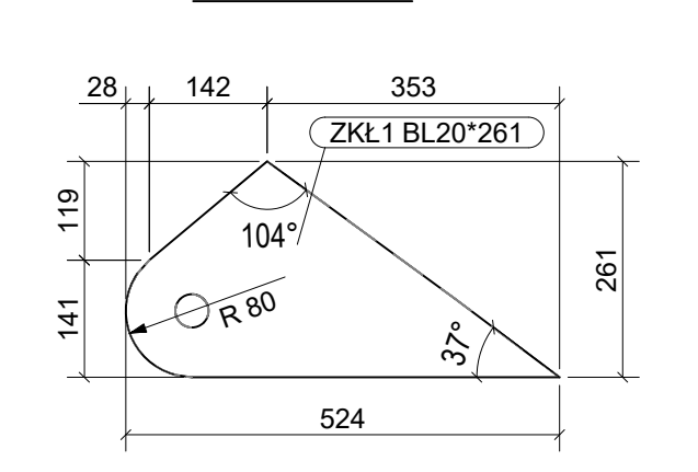
SEKCJA ŁUKU SP4 BLACHA ZAKOTWIENIA WIESZAKÓW Skala 1:10
