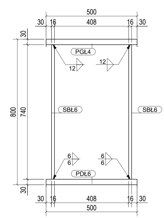
SEKCJA ŁUKU SP4 PRZEKRÓJ A-A Skala 1:10
