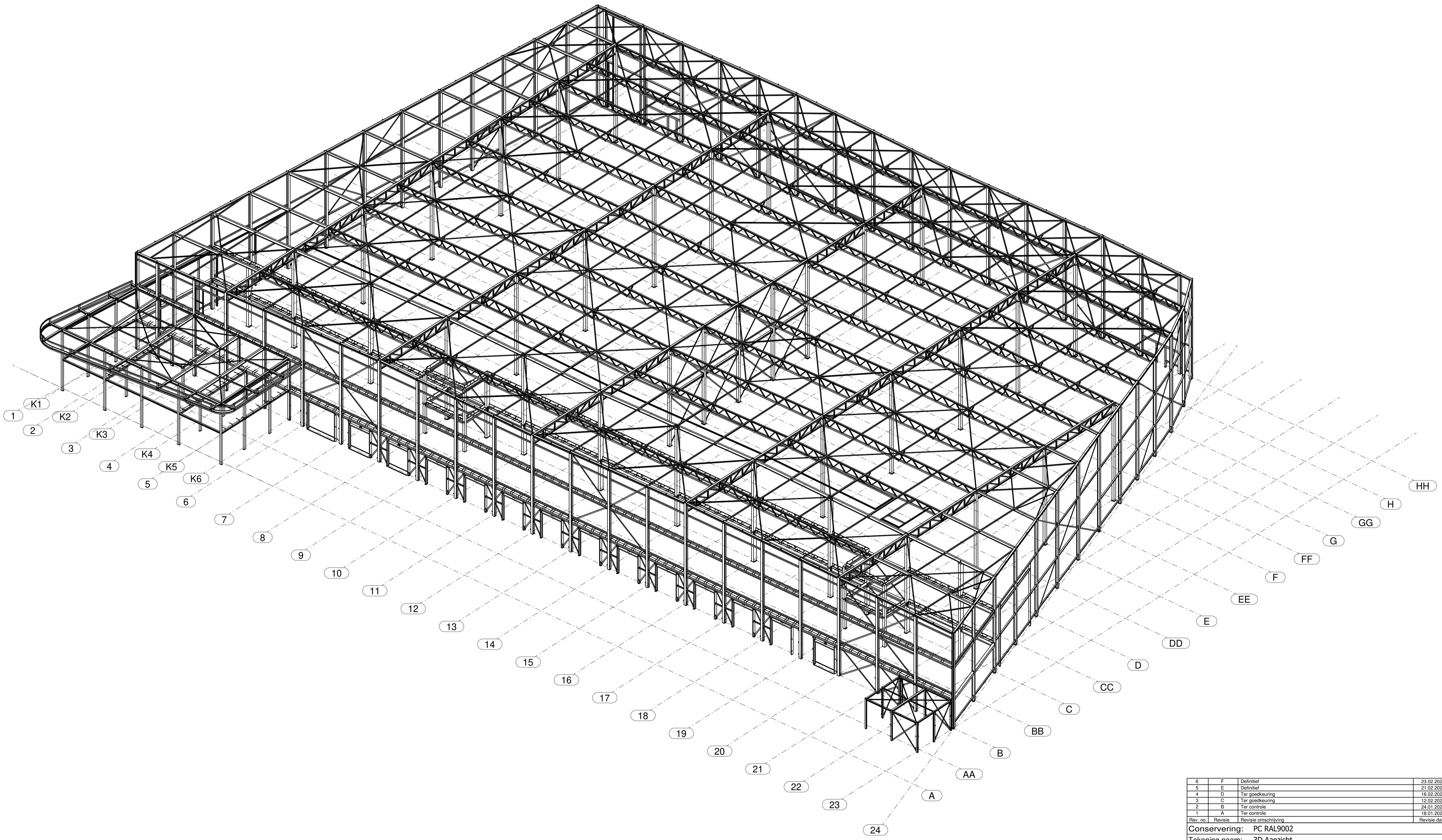
3D Overzicht 1:200
