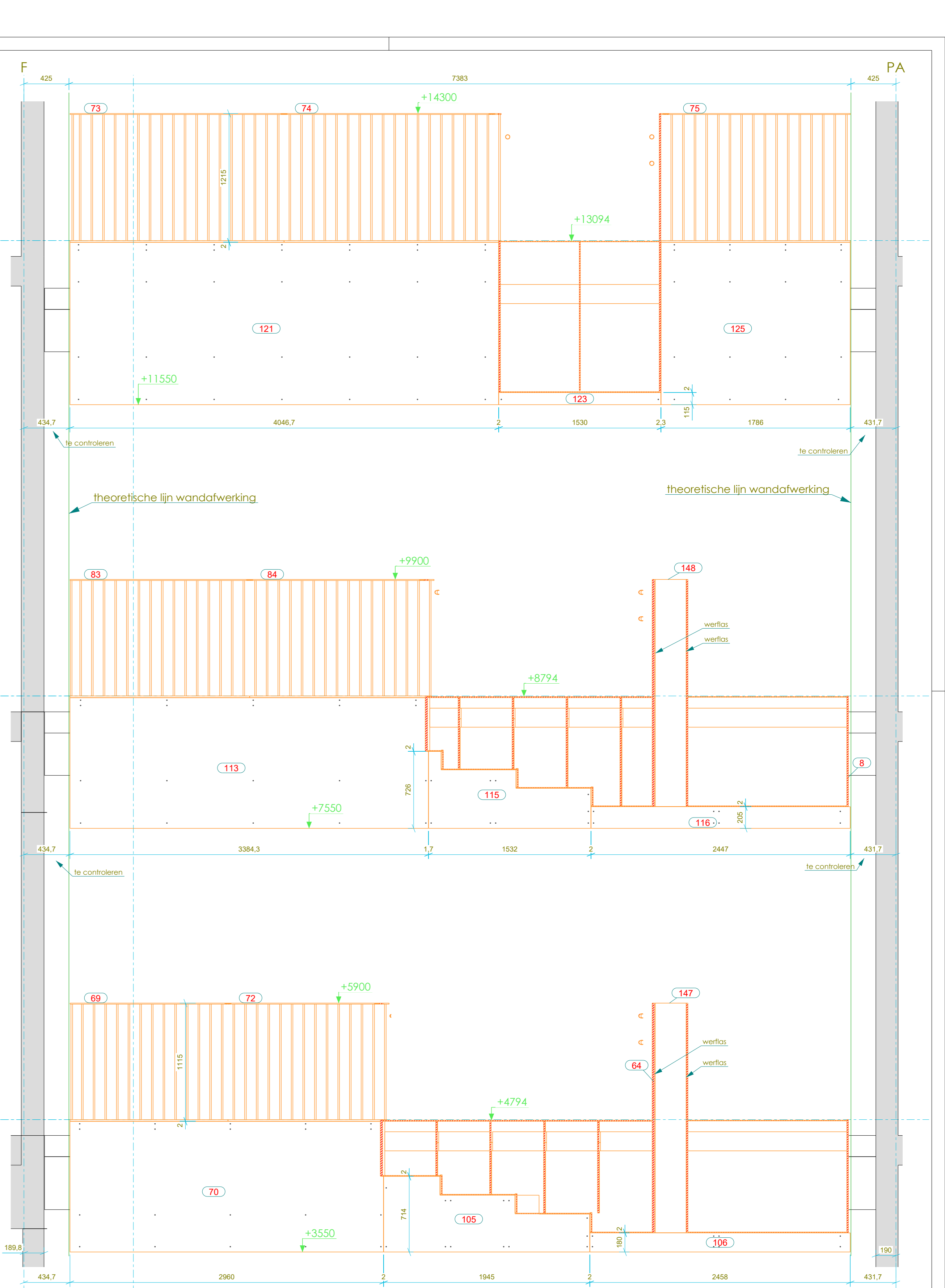
Snedes B-B 1:25
