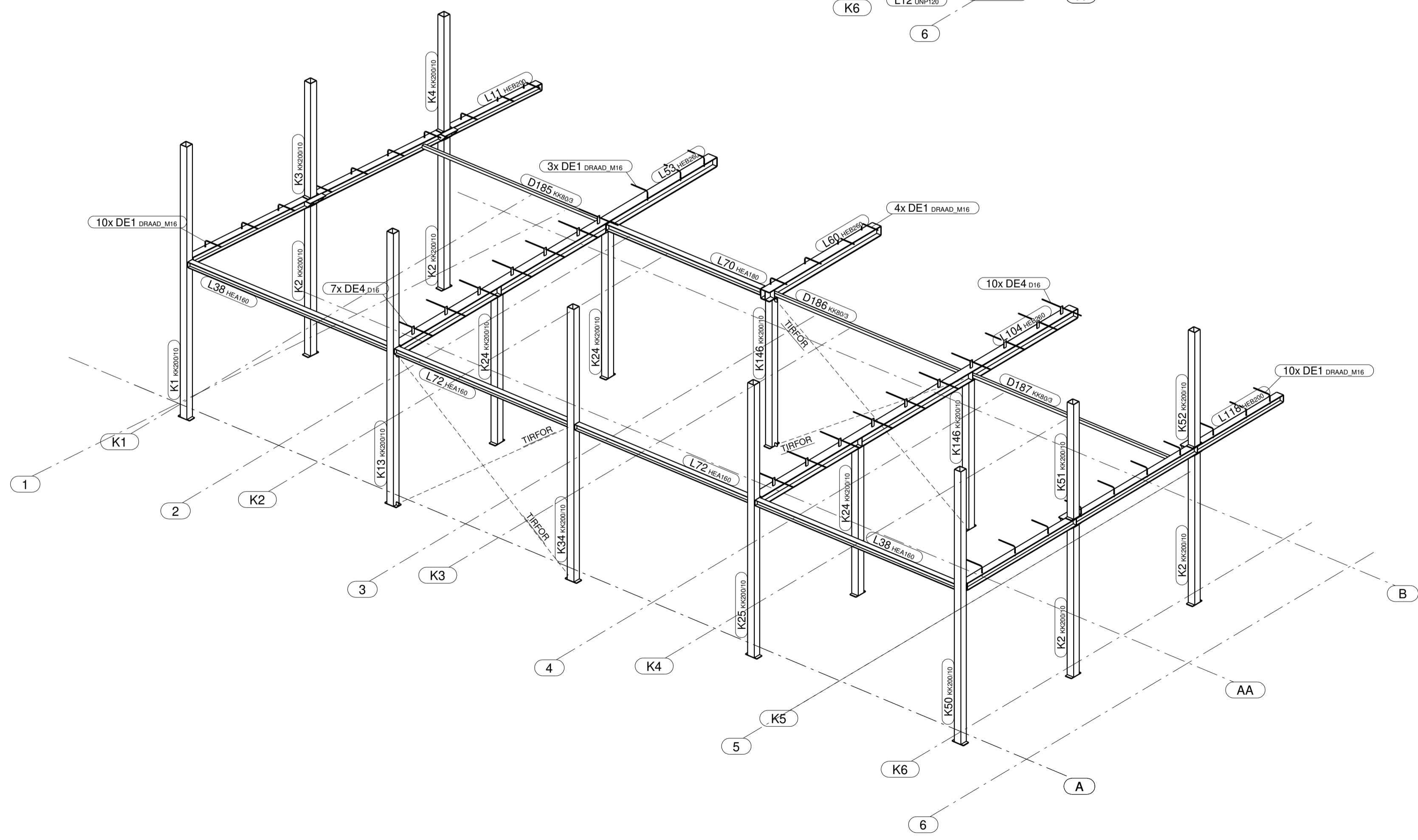
3D montage 1:75
