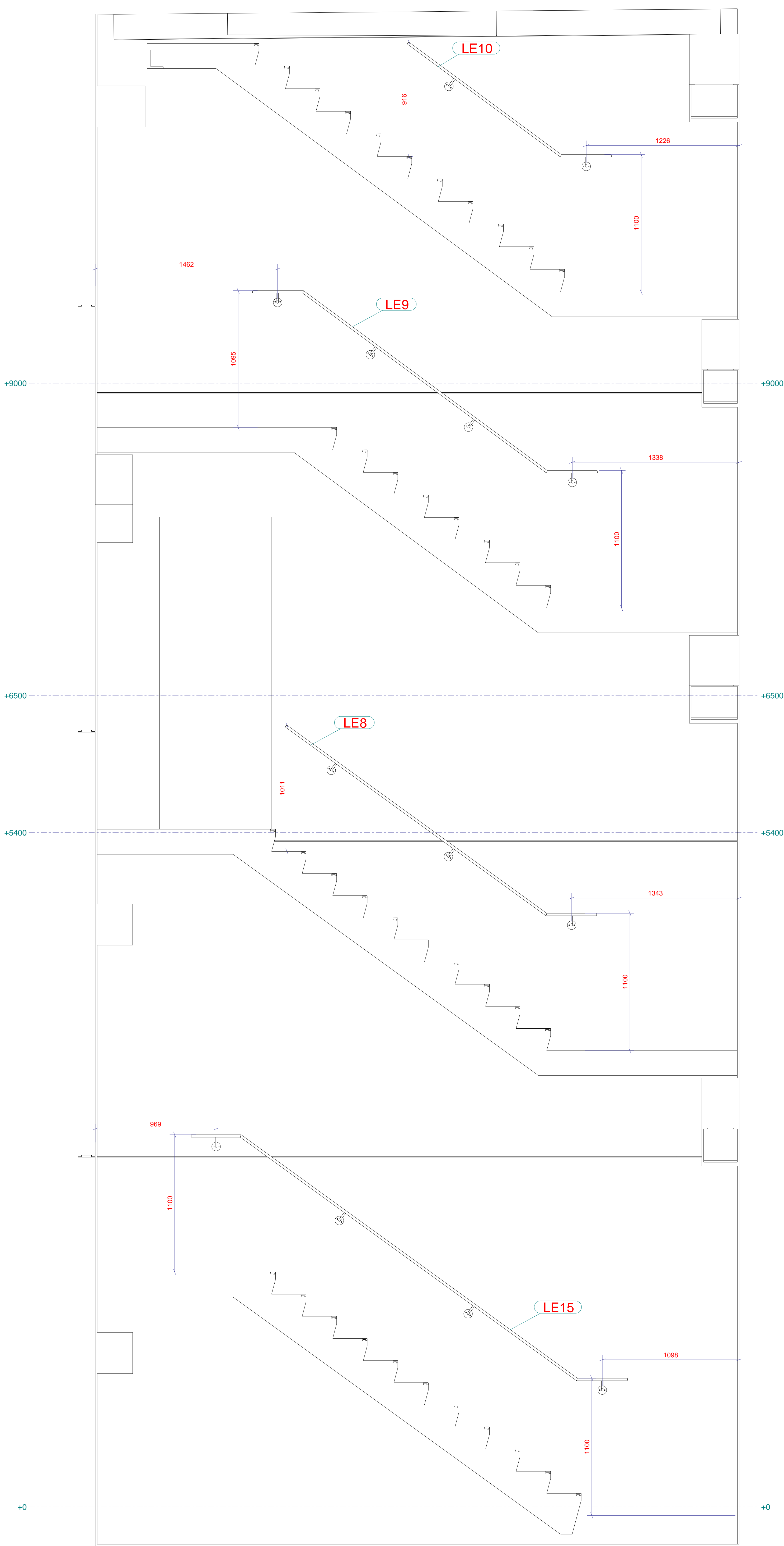
dsn B - B, 1:16
