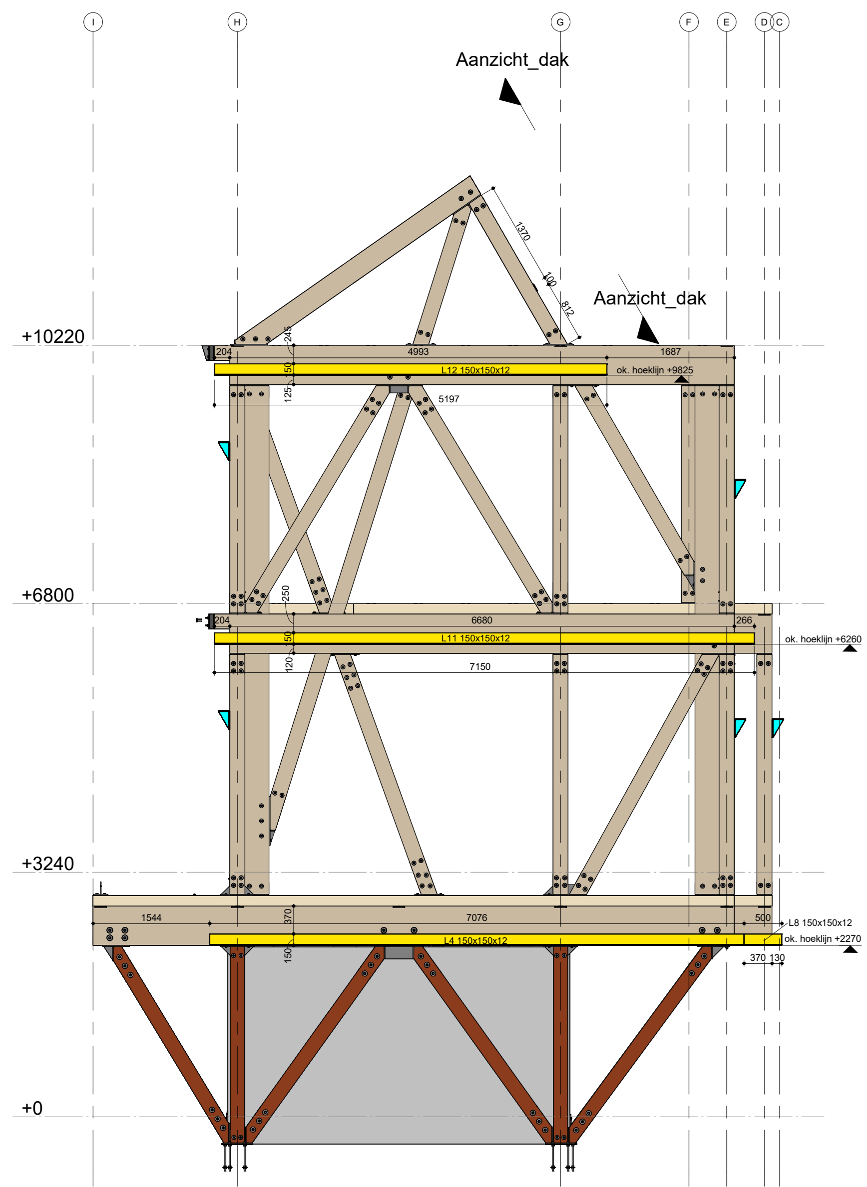
Aanzicht links
