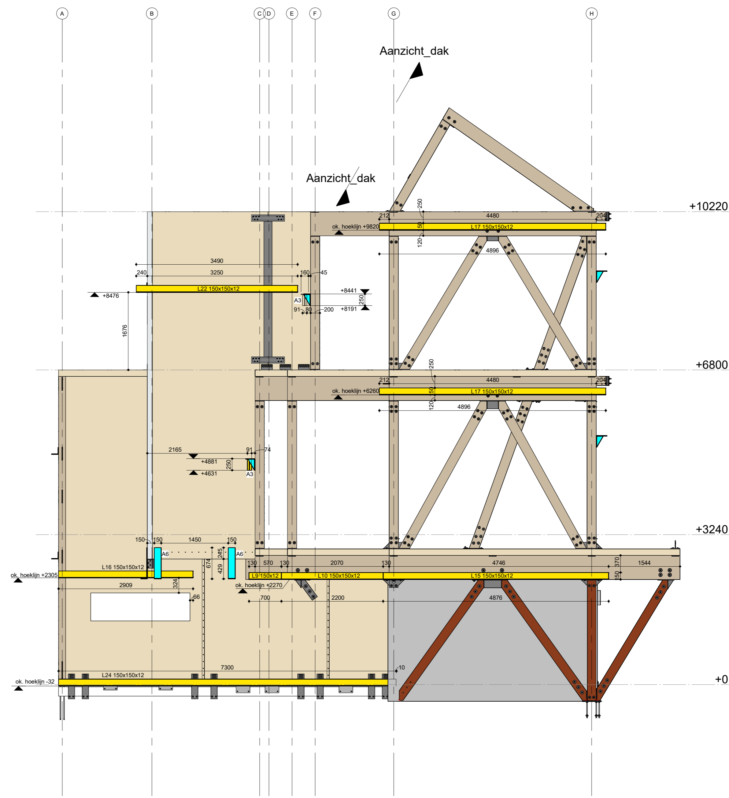
Aanzicht rechts
