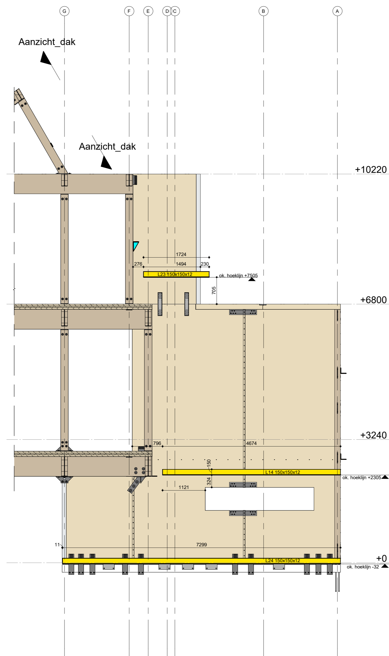
Aanzicht links1
