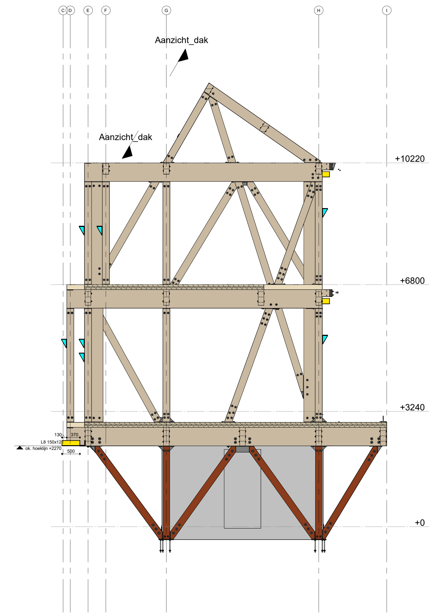
Aanzicht rechts1
