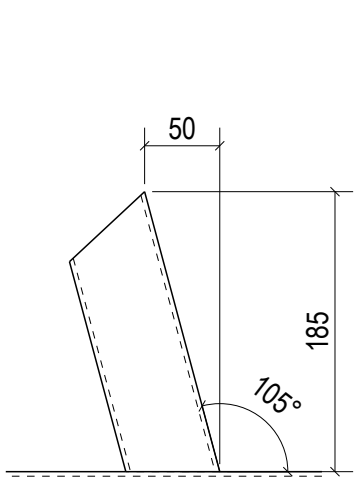
Detal A , 1:5
