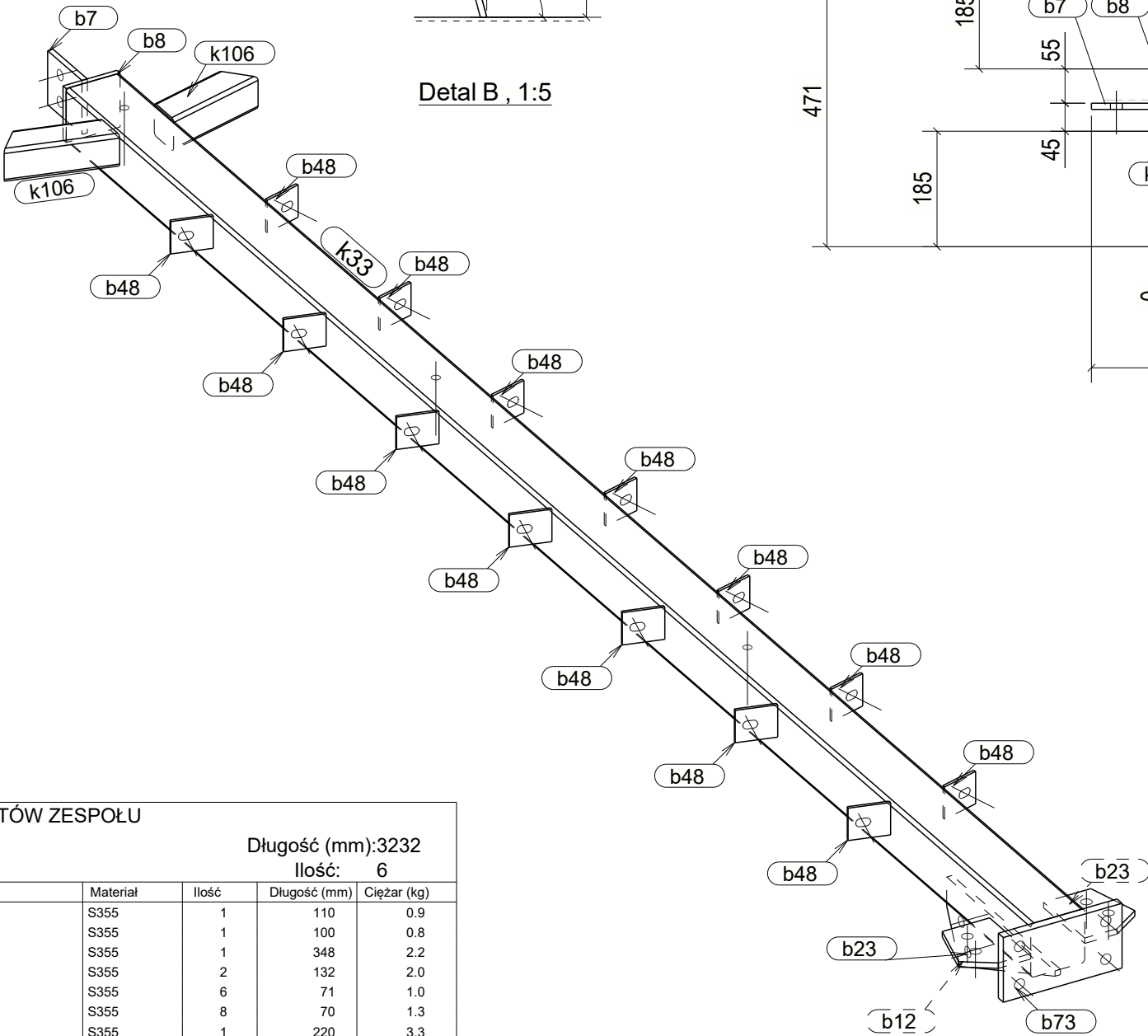
Widok 3D 1:10
