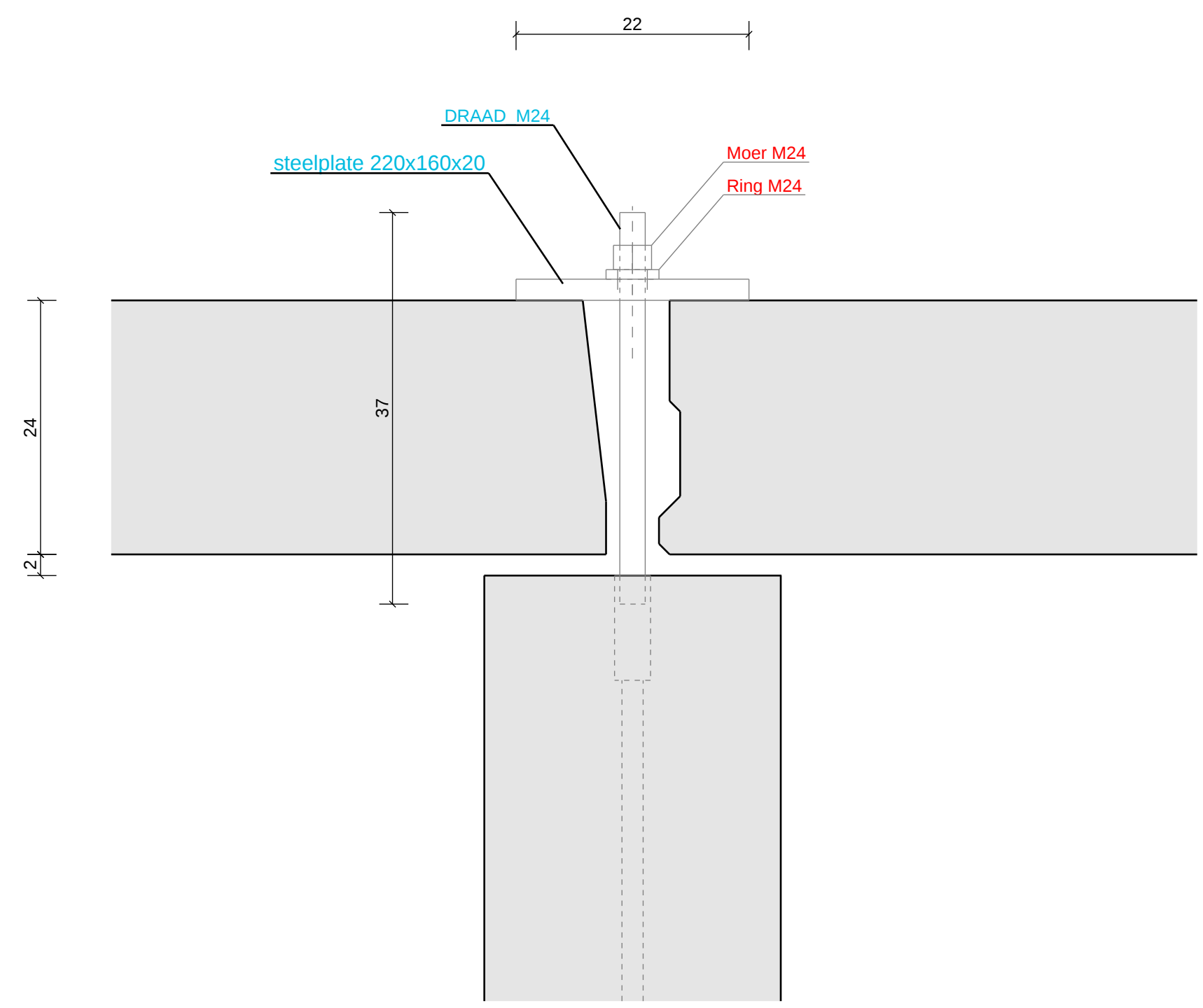
Typisch wand-vloer aansluitingsdetail
