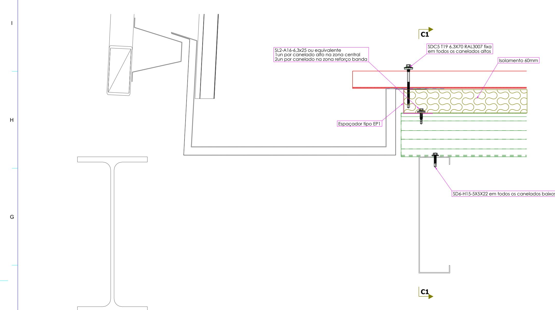
Detalhe C - Caldeiro 1:5
