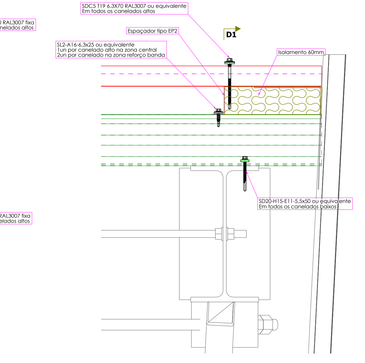
Detalhe D - Shed 1:5
