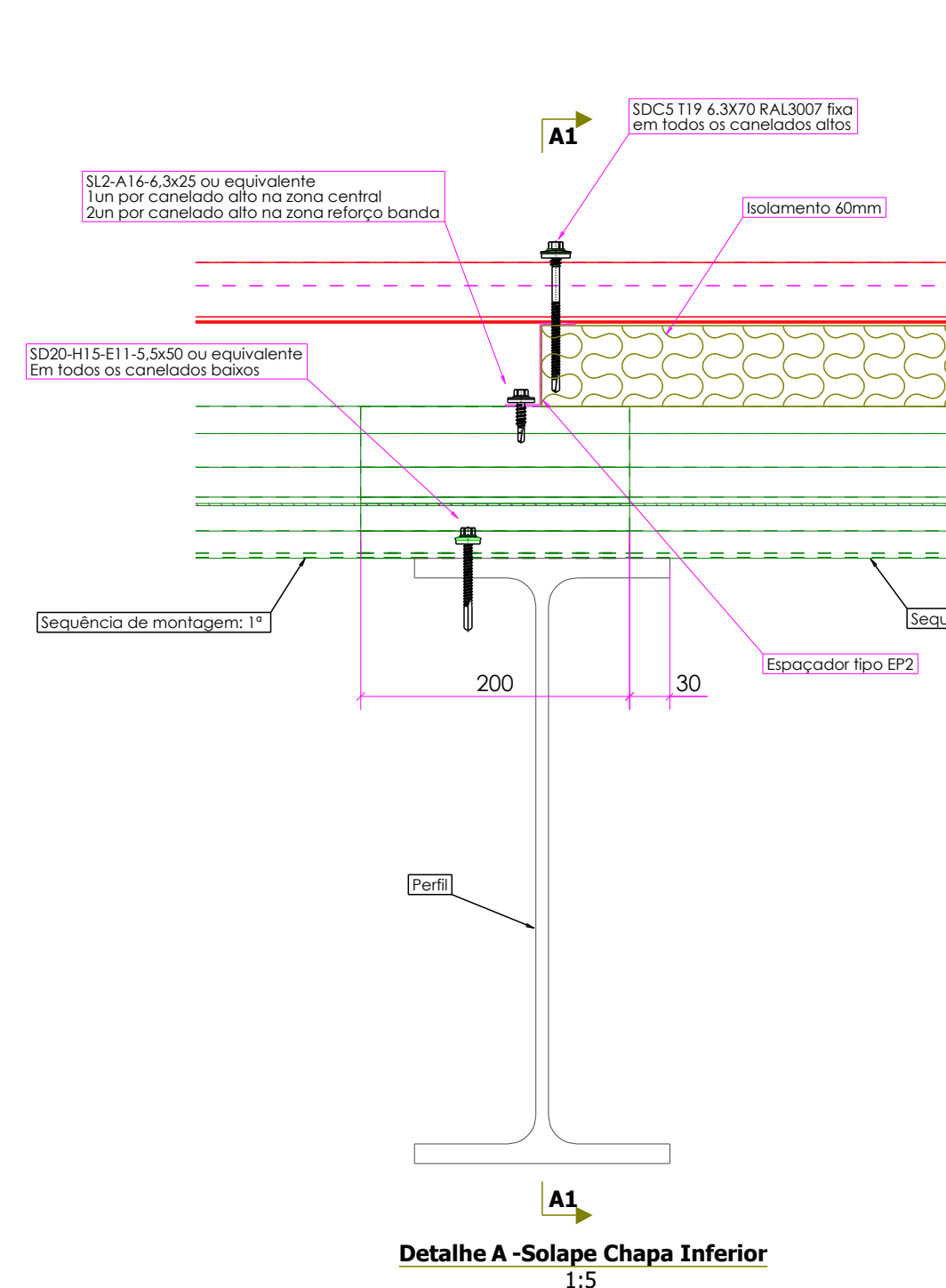
Detalhe A - Solape Chapa Inferior 1:5
