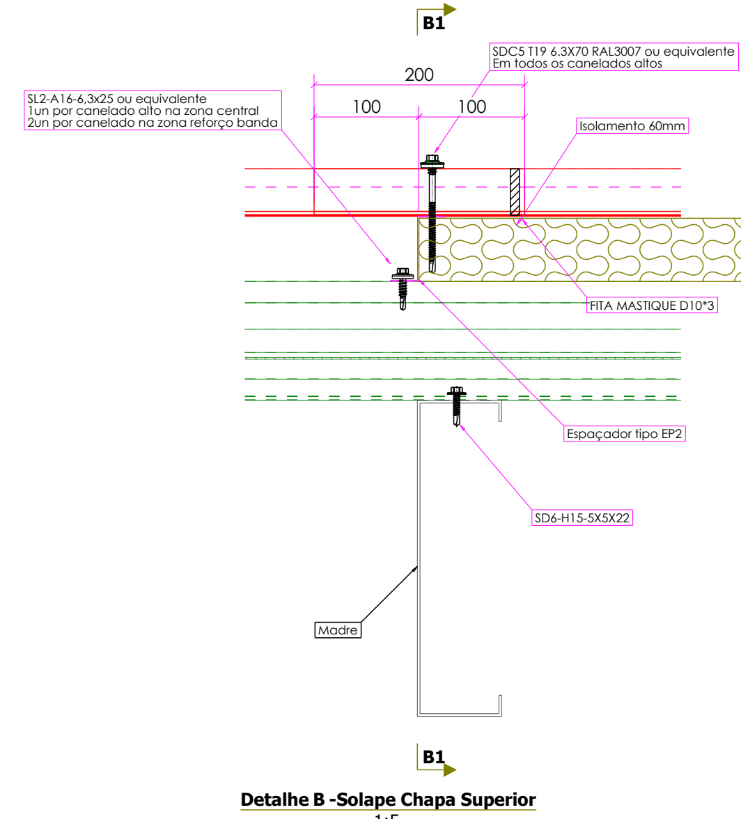
Detalhe B - Solape Chapa Superior 1:5
