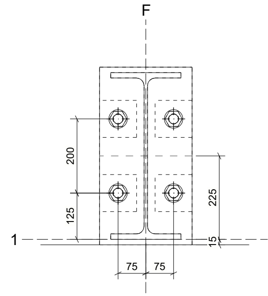
Detalhe E 1:10
