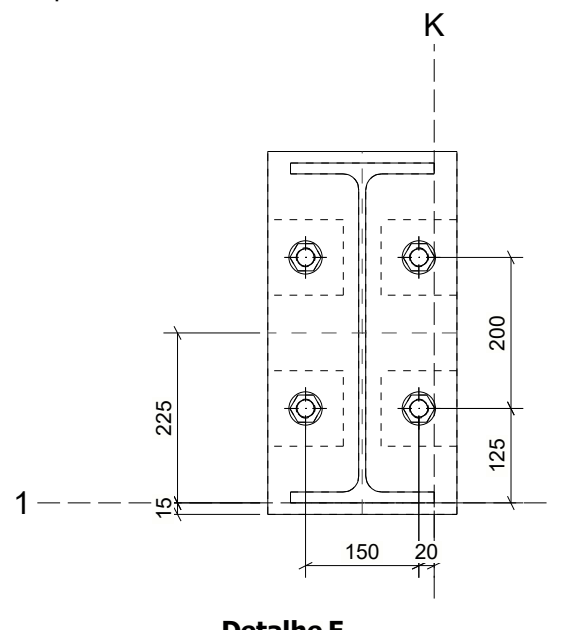
Detalhe F 1:10
