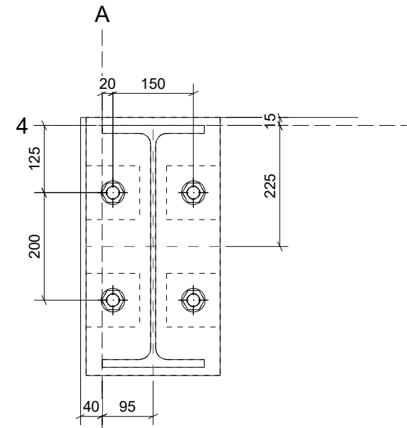
Detalhe A 1:10
