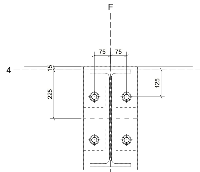
Detalhe B 1:10
