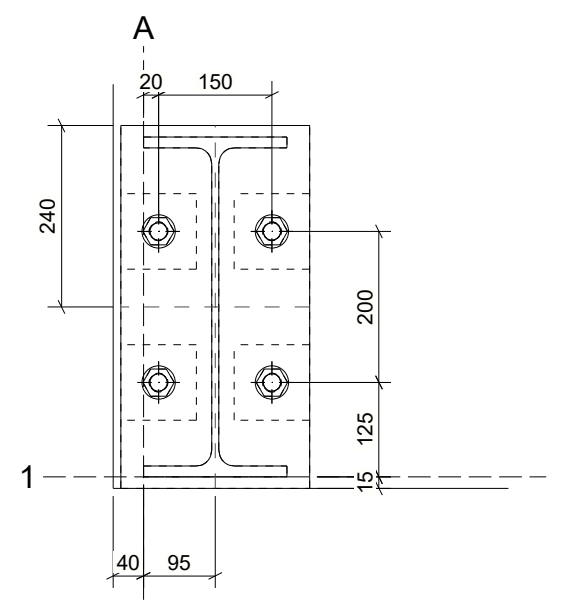
Detalhe D 1:10
