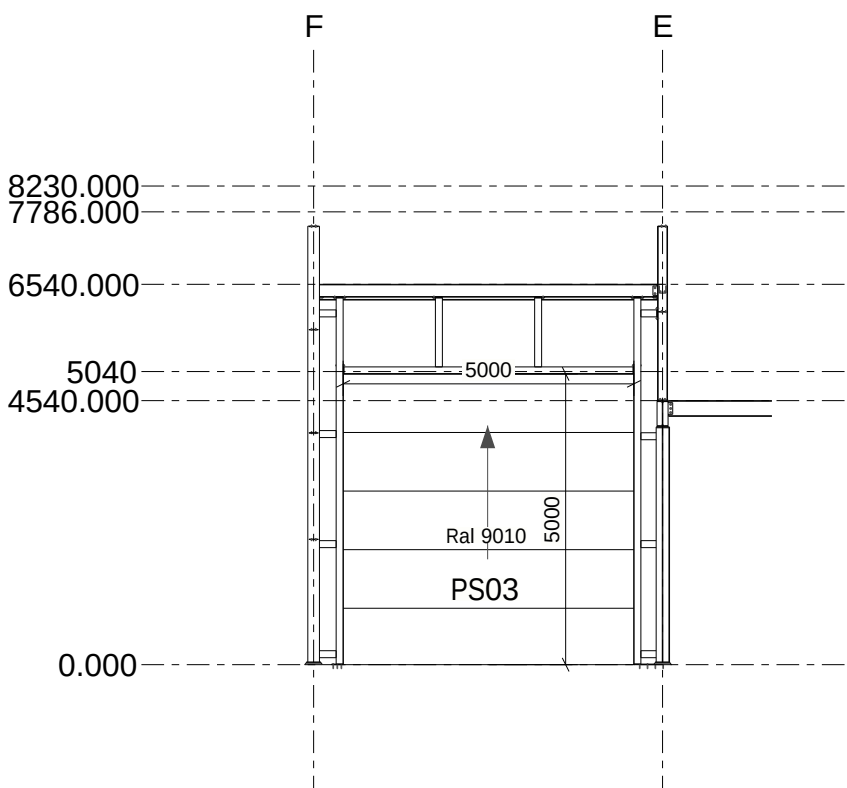
E - E
