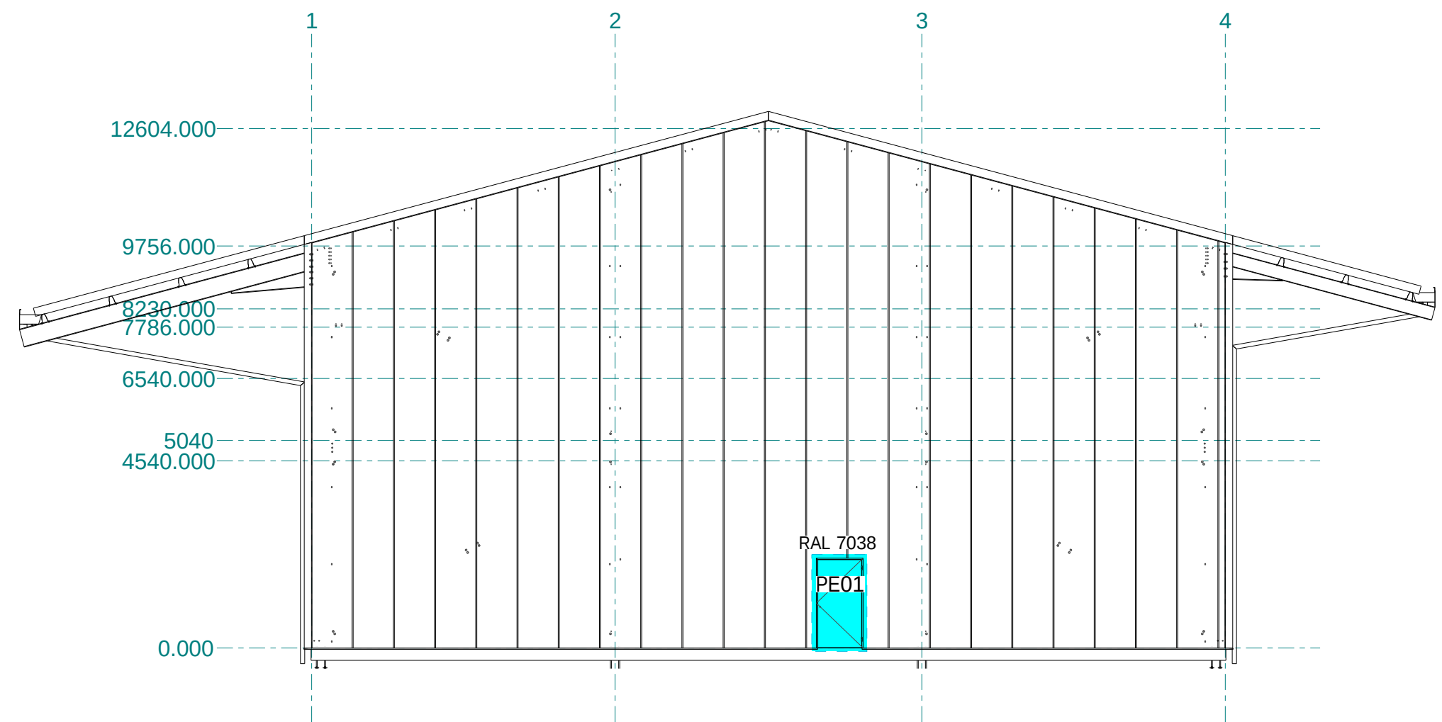
D - D
