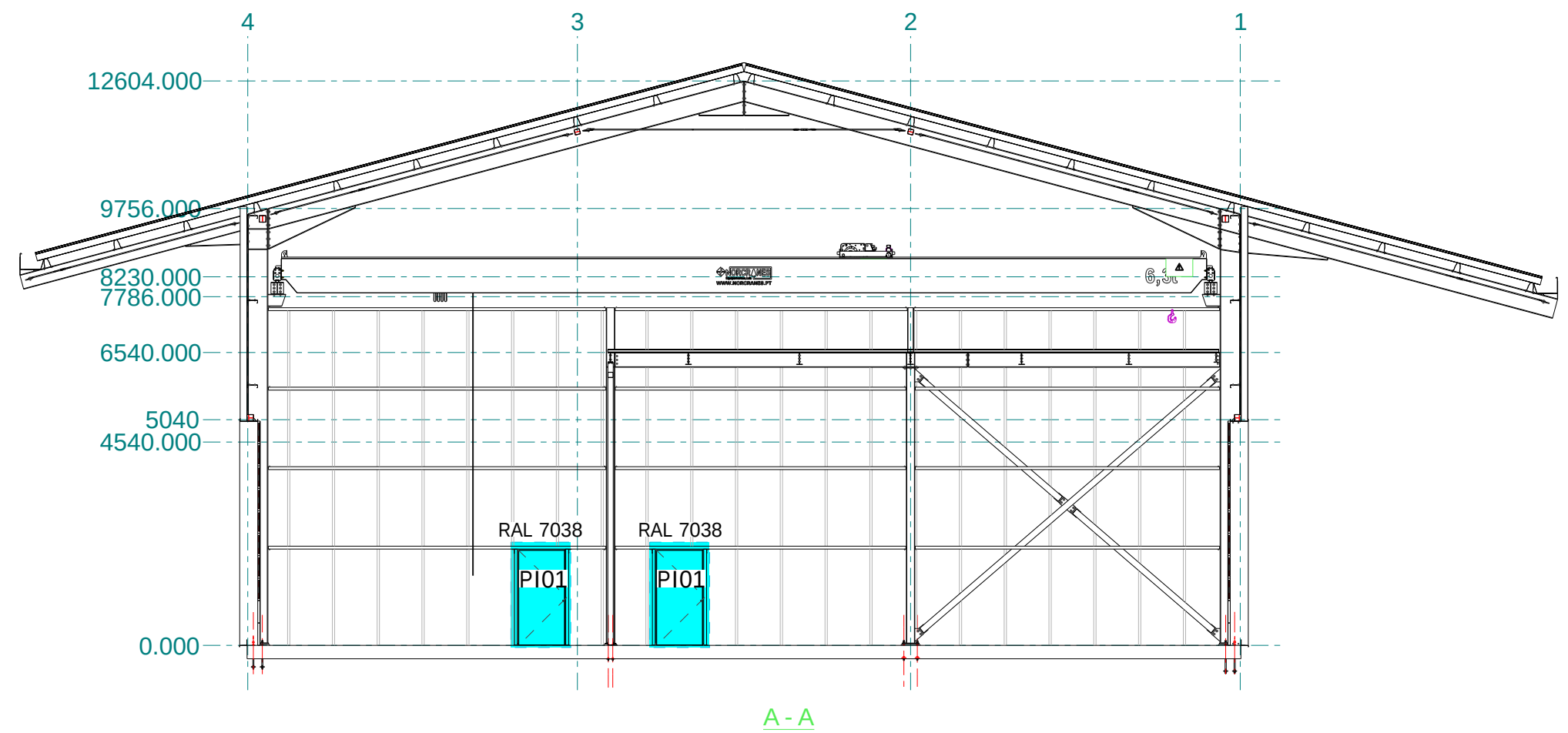
A - A
