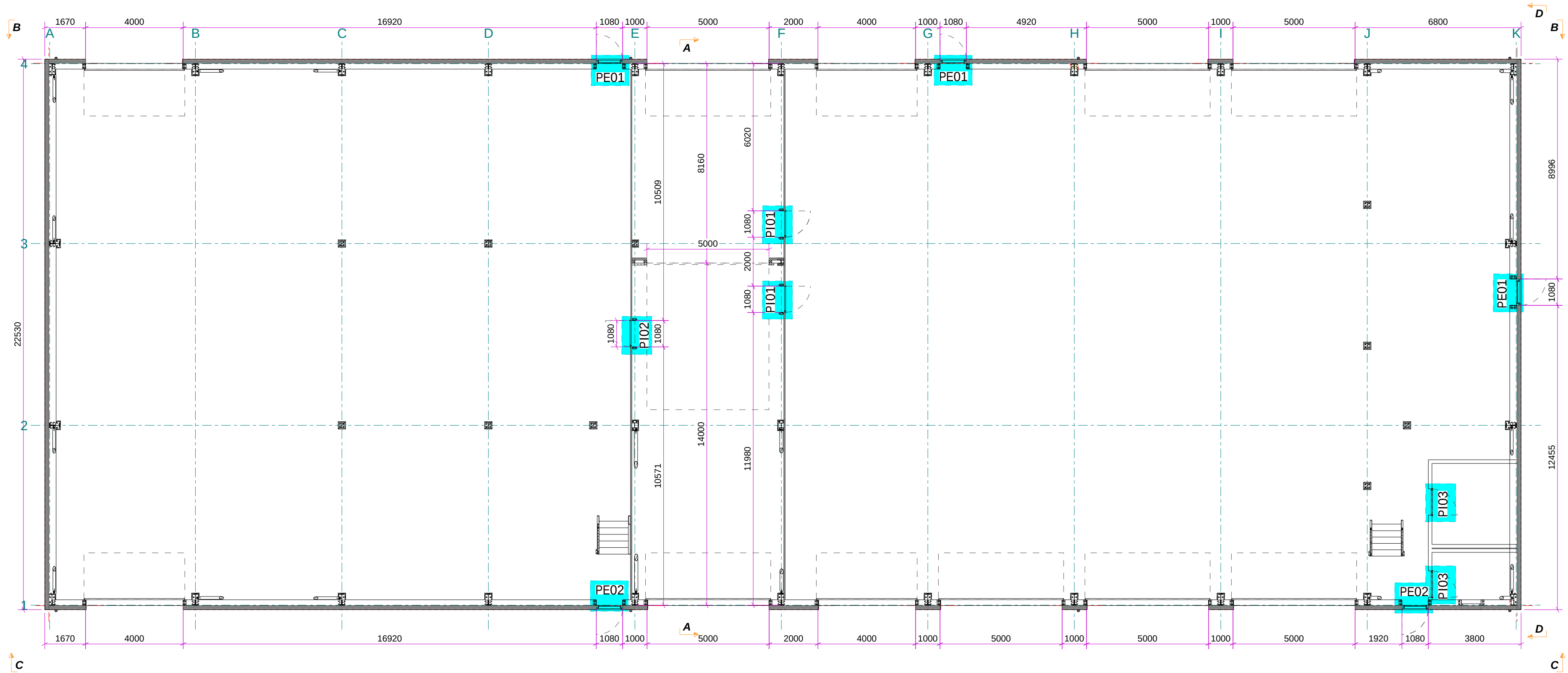
Plan Niveau +1000
