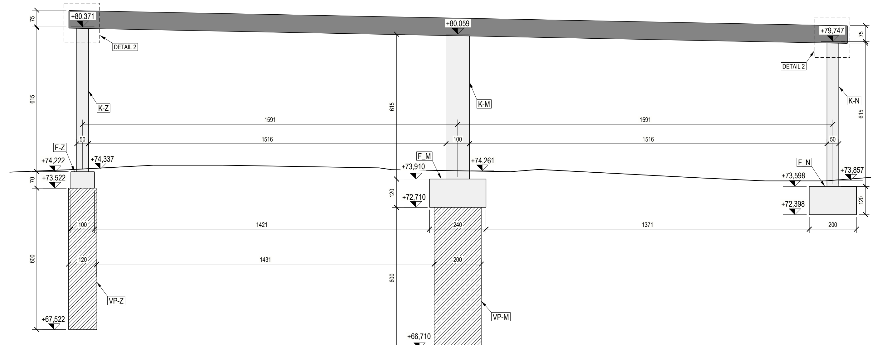
SNEDE D-D Schaal 1:100
