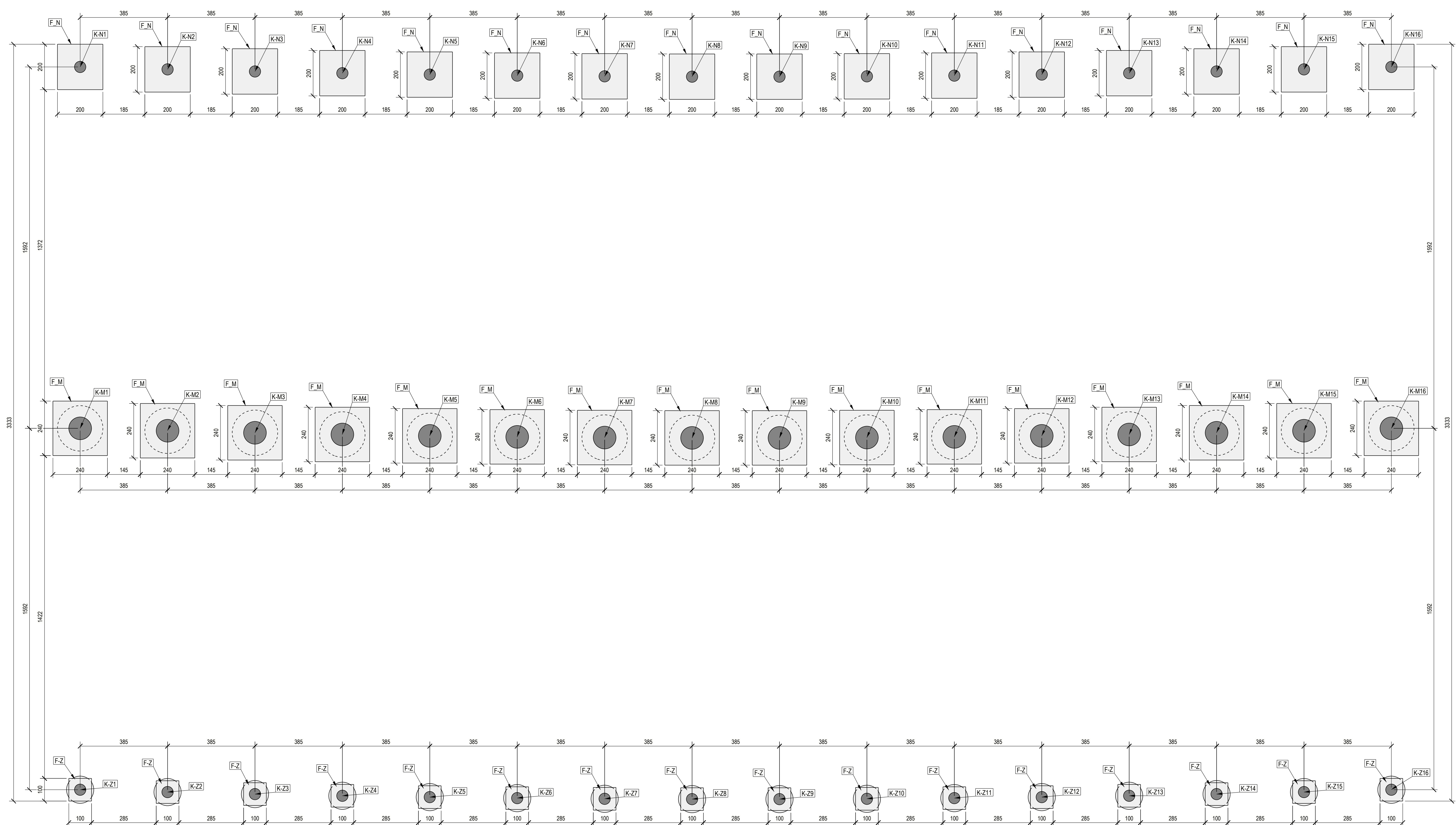
PLANZICHT FUNDERING Schaal 1:100
