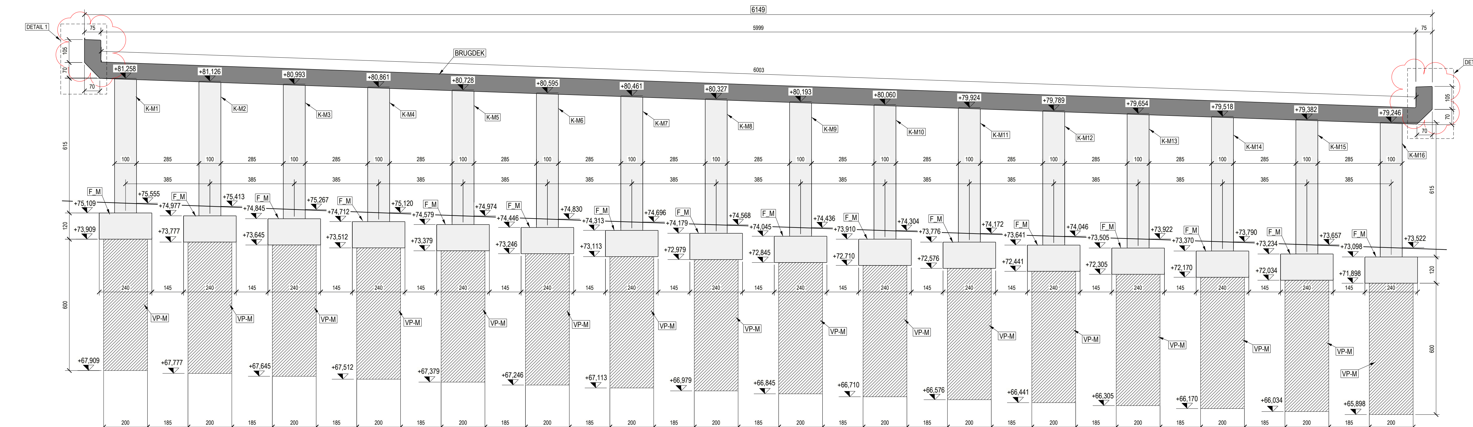
SNEDE B-B Schaal 1:100
