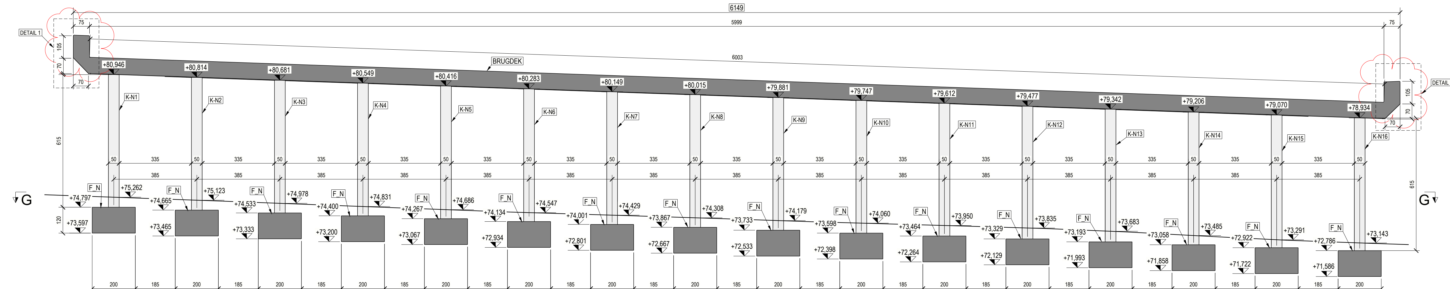
SNEDE C-C Schaal 1:100
