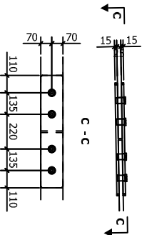
Detalhe F
