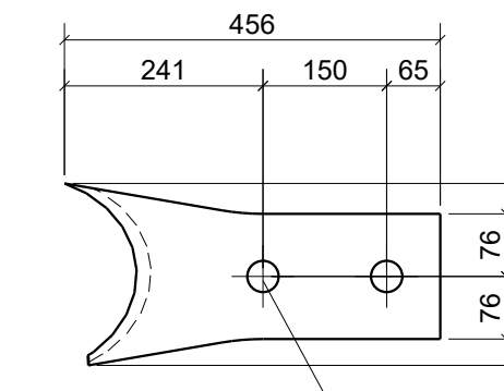
Pos. 131265 Stk. 2 Stahl S355J2
