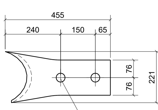
Pos. 131215 Stk. 2 Stahl S355J2
