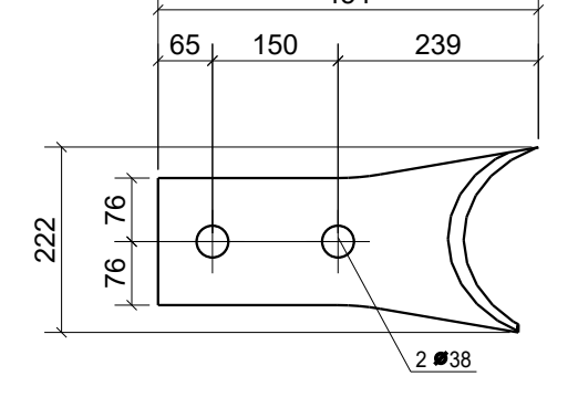
Pos. 131257 Stk. 2 Stahl S355J2
