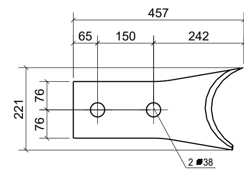
Pos. 131204 Stk. 2 Stahl S355J2
