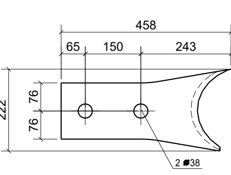
Pos. 131287 Stk. 2 Stahl S355J2
