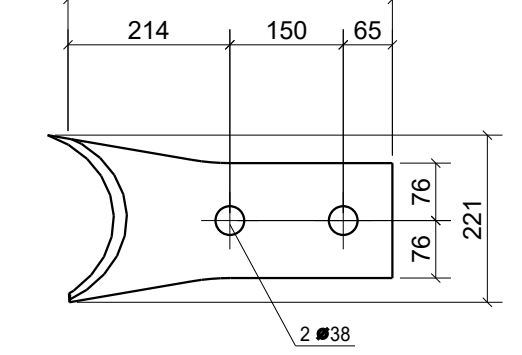
Pos. 131260 Stk. 2 Stahl S355J2
