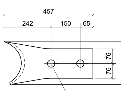
Pos. 131290 Stk. 2 Stahl S355J2
