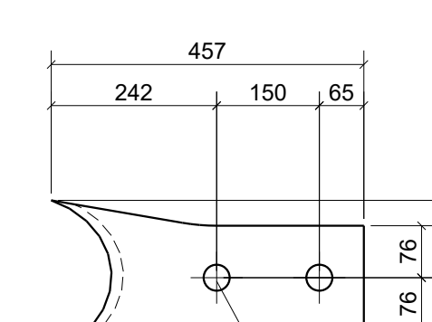
Pos. 131272 Stk. 2 Stahl S355J2
