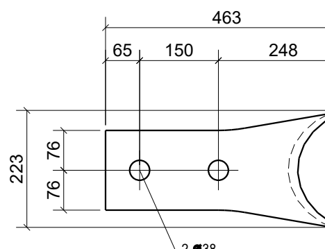
Pos. 131281 Stk. 2 Stahl S355J2
