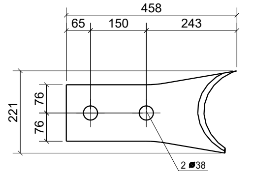
Pos. 131216 Stk. 2 Stahl S355J2
