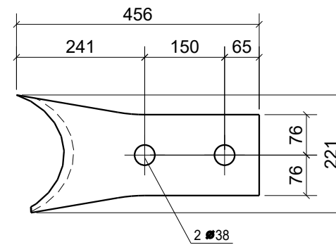
Pos. 131271 Stk. 2 Stahl S355J2
