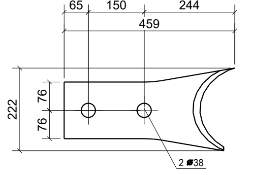
Pos. 131221 Stk. 2 Stahl S355J2
