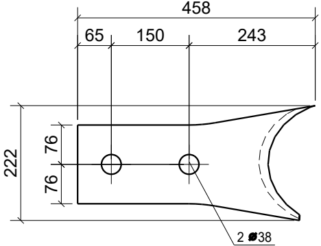
Pos. 131207 Stk. 2 Stahl S355J2
