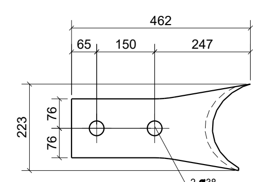
Pos. 131258 Stk. 2 Stahl S355J2
