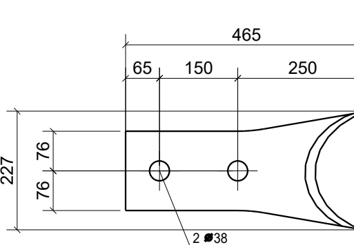
Pos. 131228 Stk. 2 Stahl S355J2
