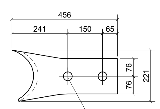
Pos. 131259 Stk. 2 Stahl S355J2
