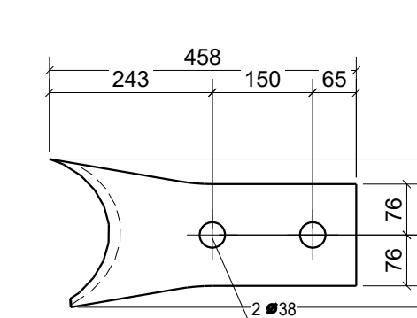
Pos. 131289 Stk. 2 Stahl S355J2
