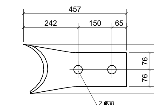
Pos. 131220 Stk. 2 Stahl S355J2
