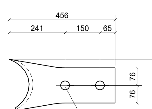
Pos. 131201 Stk. 2 Stahl S355J2
