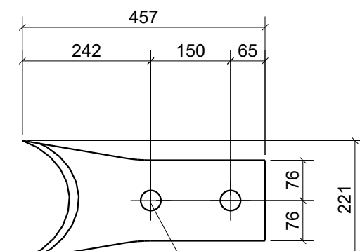
Pos. 131279 Stk. 2 Stahl S355J2
