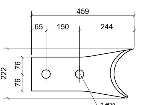
Pos. 131209 Stk. 2 Stahl S355J2
