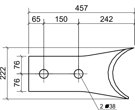
Pos. 131223 Stk. 2 Stahl S355J2
