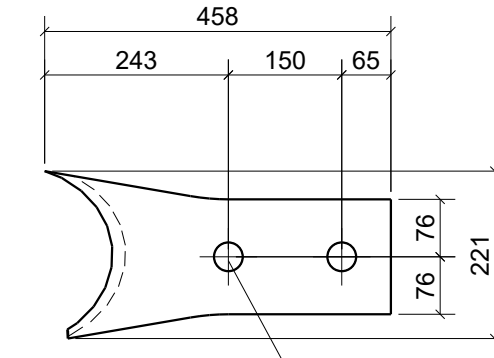
Pos. 131200 Stk. 2 Stahl S355J2
