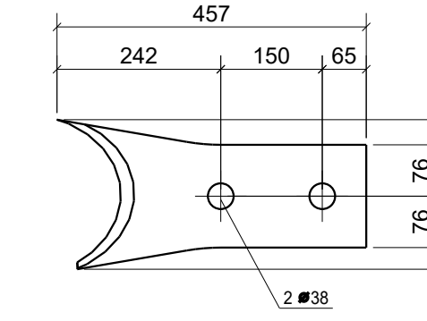
Pos. 131273 Stk. 2 Stahl S355J2
