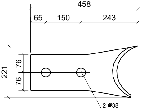
Pos. 131218 Stk. 2 Stahl S355J2
