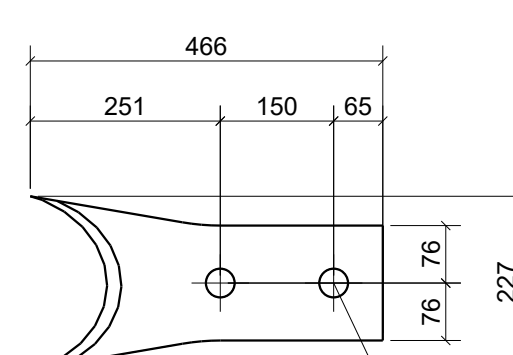
Pos. 131227 Stk. 2 Stahl S355J2
