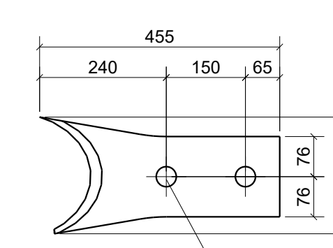
Pos. 131276 Stk. 2 Stahl S355J2
