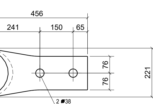
Pos. 131256 Stk. 2 Stahl S355J2
