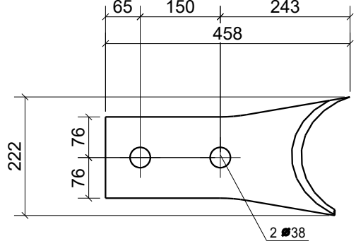
Pos. 131212 Stk. 2 Stahl S355J2
