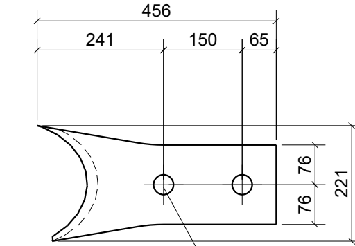
Pos. 131280 Stk. 2 Stahl S355J2
