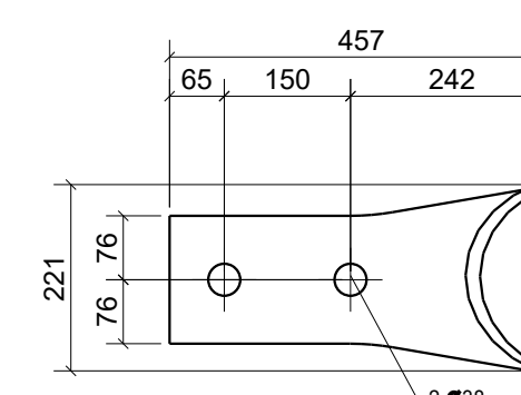
Pos. 131283 Stk. 2 Stahl S355J2
