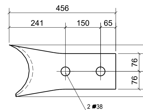
Pos. 131268 Stk. 2 Stahl S355J2
