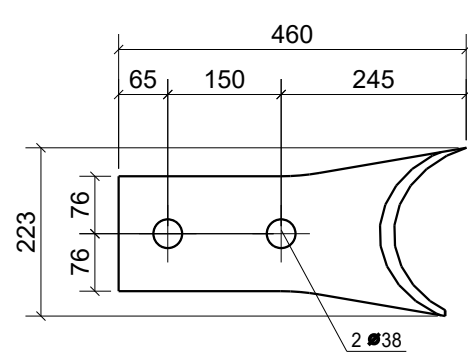
Pos. 131278 Stk. 2 Stahl S355J2
