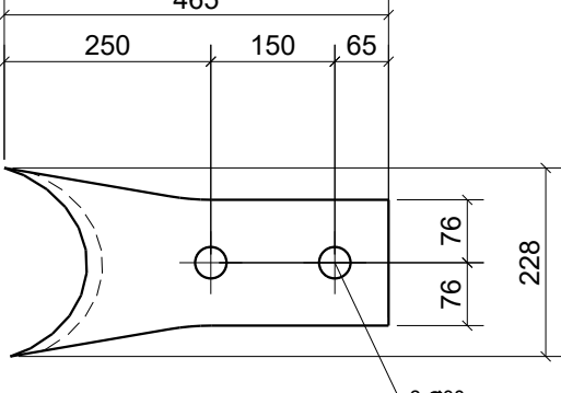
Pos. 131226 Stk. 2 Stahl S355J2
