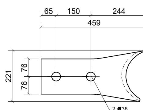
Pos. 131270 Stk. 2 Stahl S355J2
