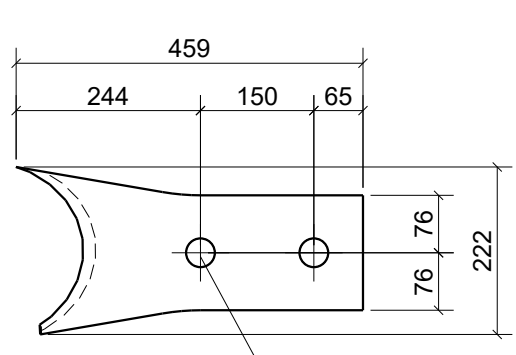
Pos. 131219 Stk. 2 Stahl S355J2
