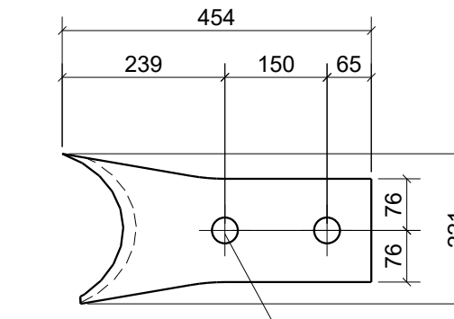
Pos. 131211 Stk. 2 Stahl S355J2
