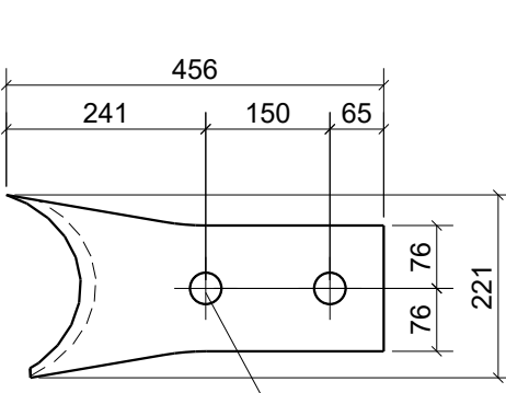
Pos. 131262 Stk. 2 Stahl S355J2
