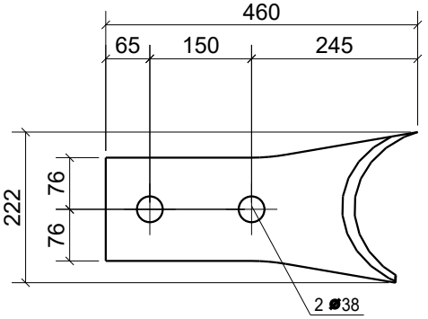
Pos. 131275 Stk. 2 Stahl S355J2
