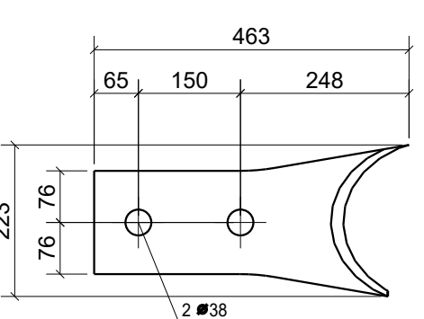
Pos. 131291 Stk. 2 Stahl S355J2
