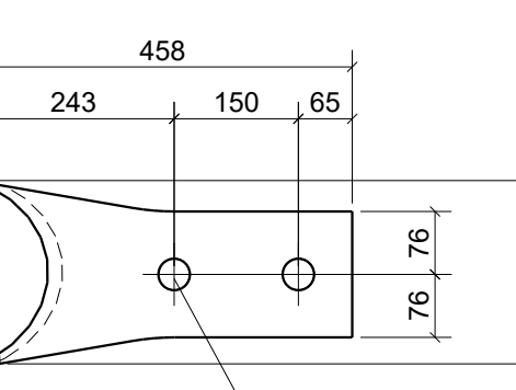
Pos. 131288 Stk. 2 Stahl S355J2
