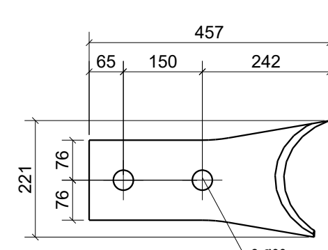
Pos. 131286 Stk. 2 Stahl S355J2
