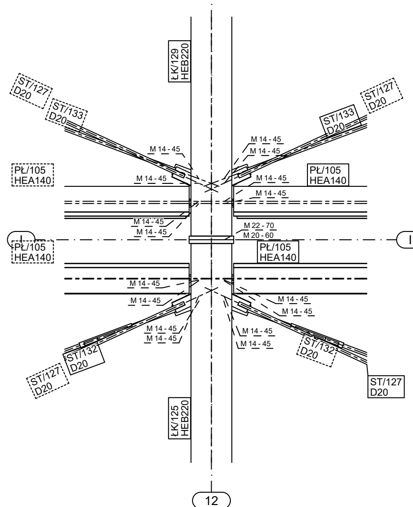
DETAL B SKALA : 1:20
