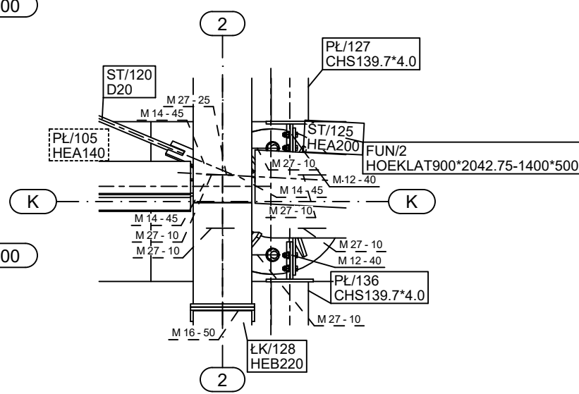
DETAL D SKALA : 1:20
