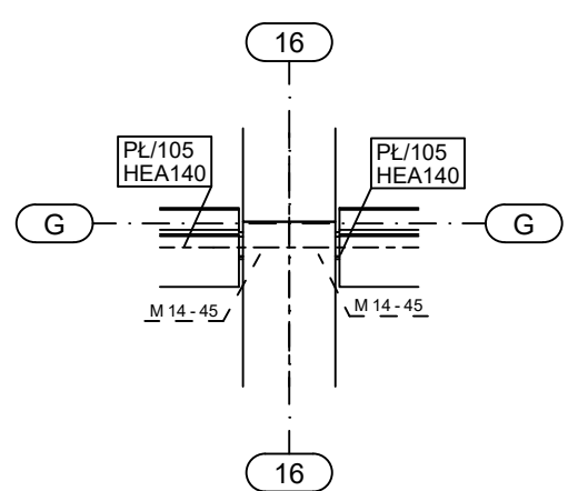
DETAL D SKALA : 1:20
