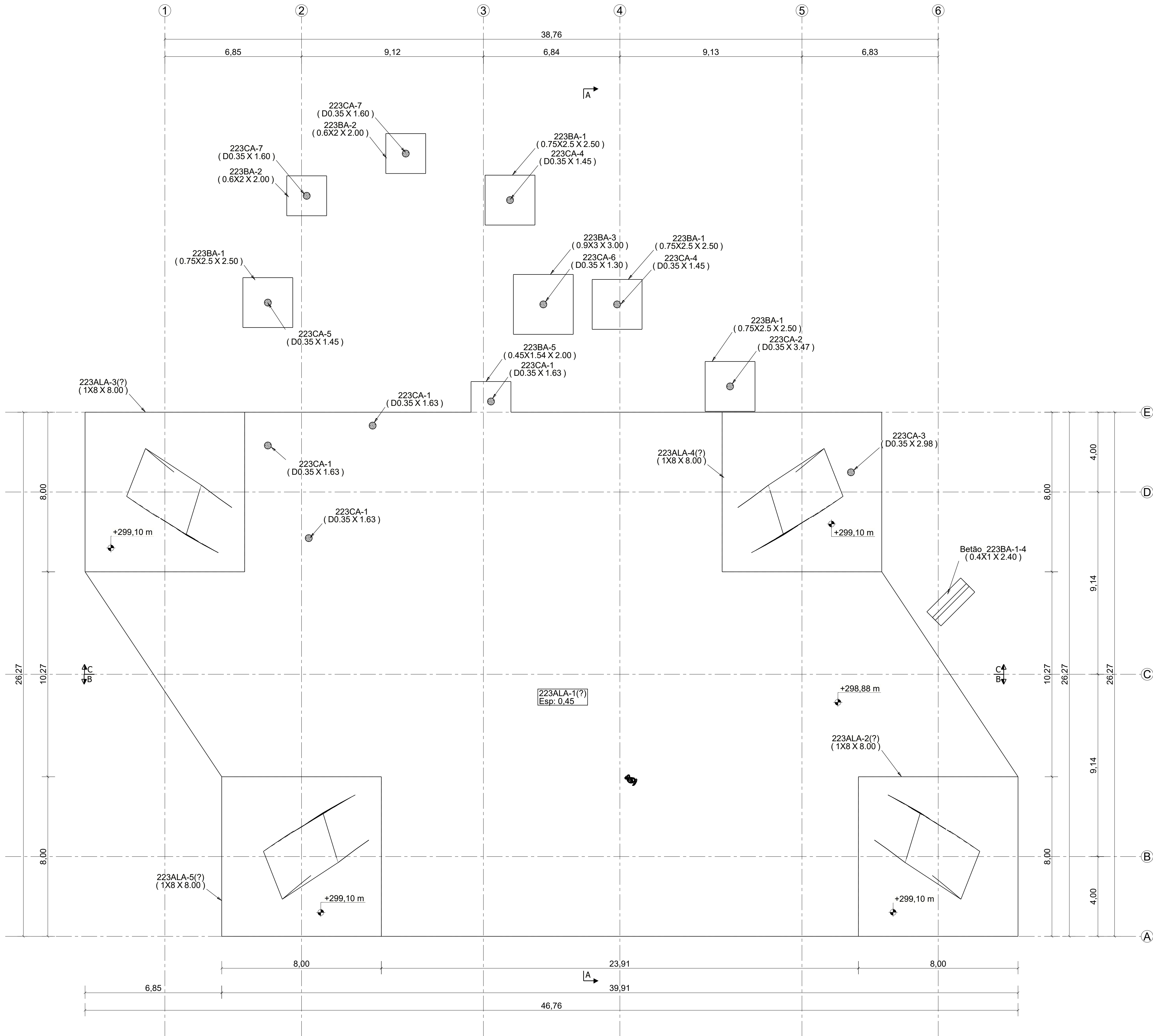
Planta | Nível 299.10 1:100
