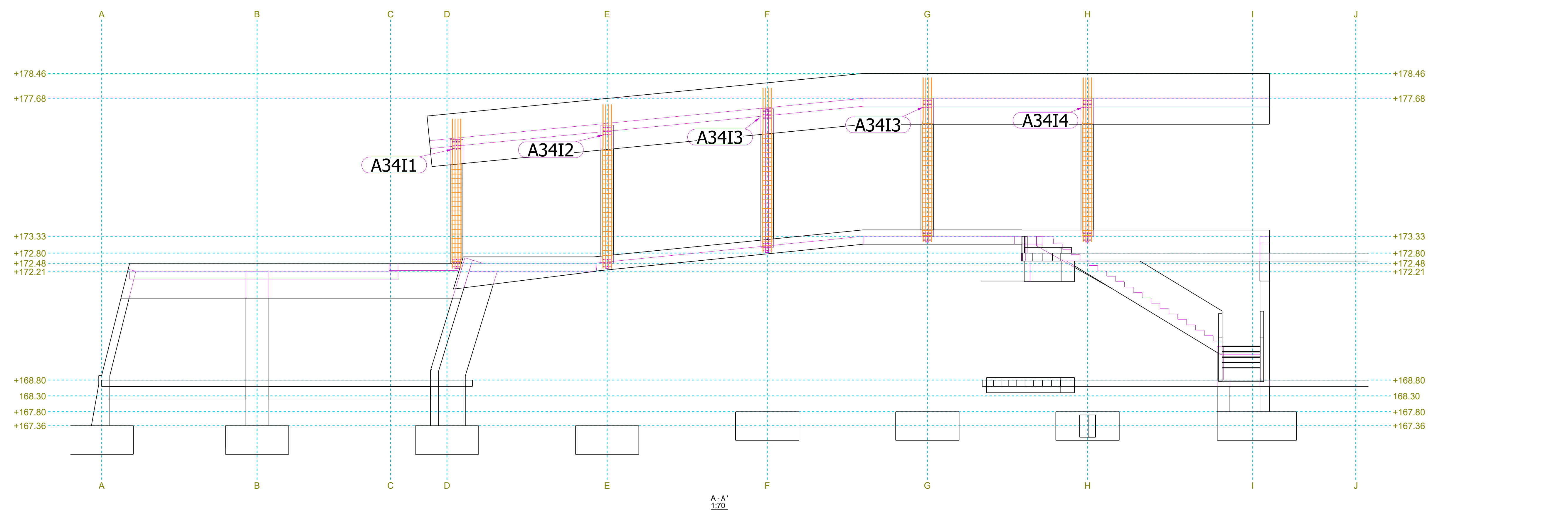
A-A 1:20
