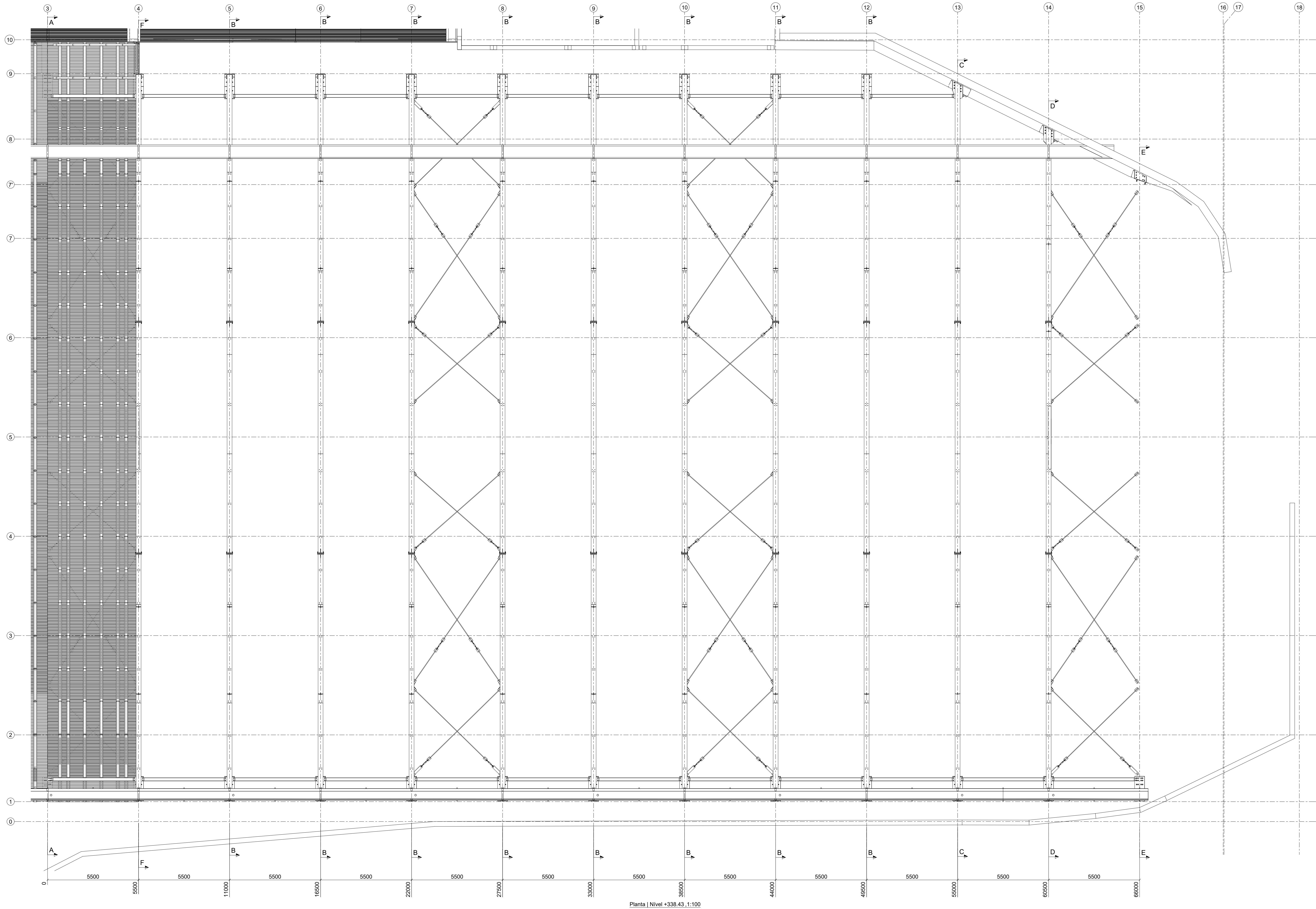
Planta | Nivel +338.43 | 1:100
