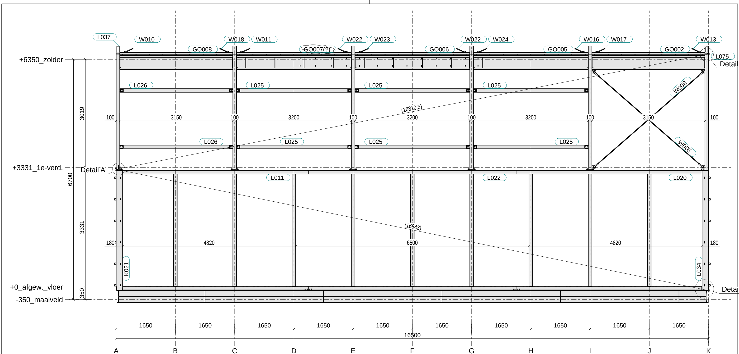
Aanzicht as 5-1 Schaal 1:50
