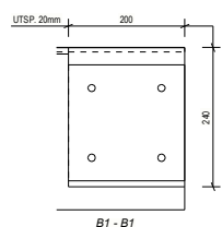
B1-B1 1:5
