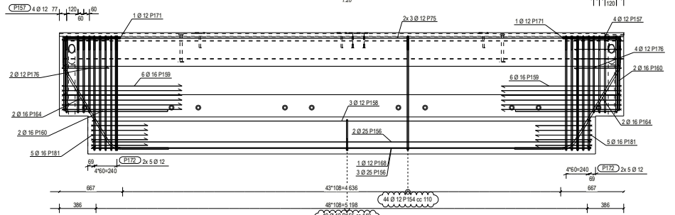
OPPRISS OPP I FORM 1:20
