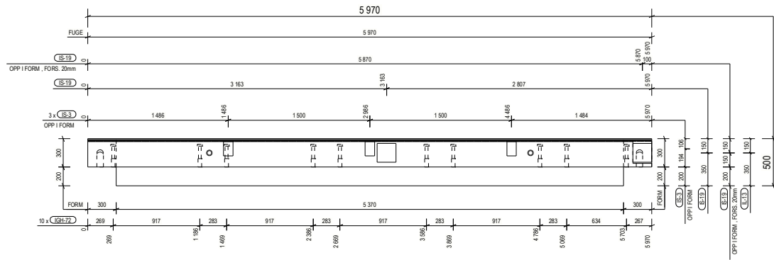
OPPRISS OPP I FORM 1:20
