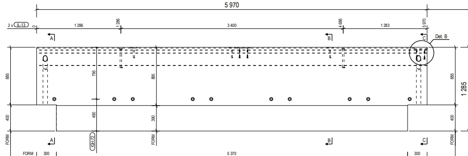
OPPRISS OPP I FORM 1:20
