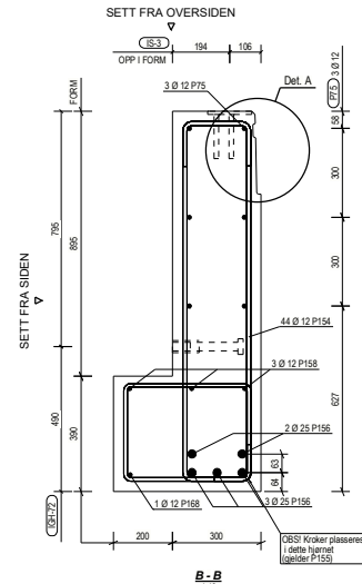
B-B 1:10
