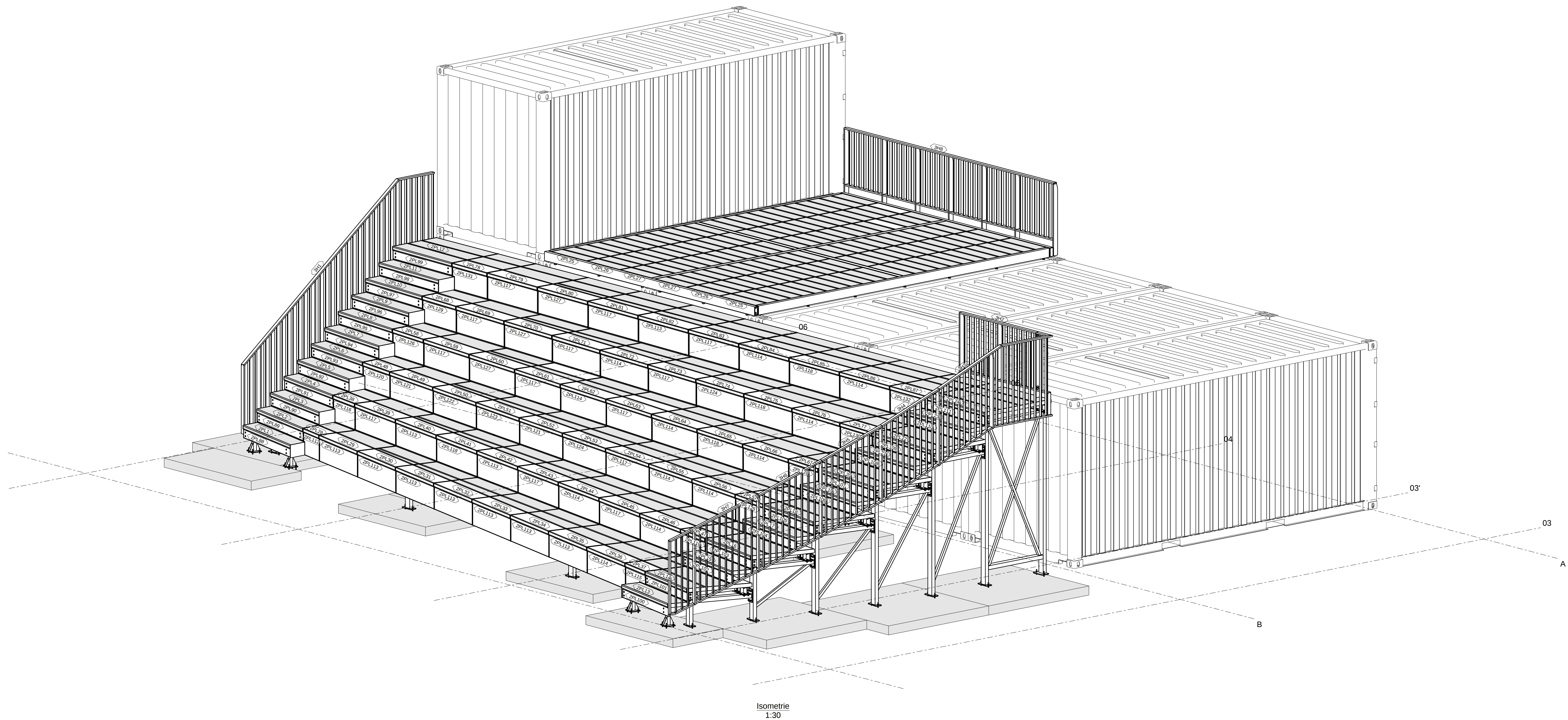
Isometrie 1:30
