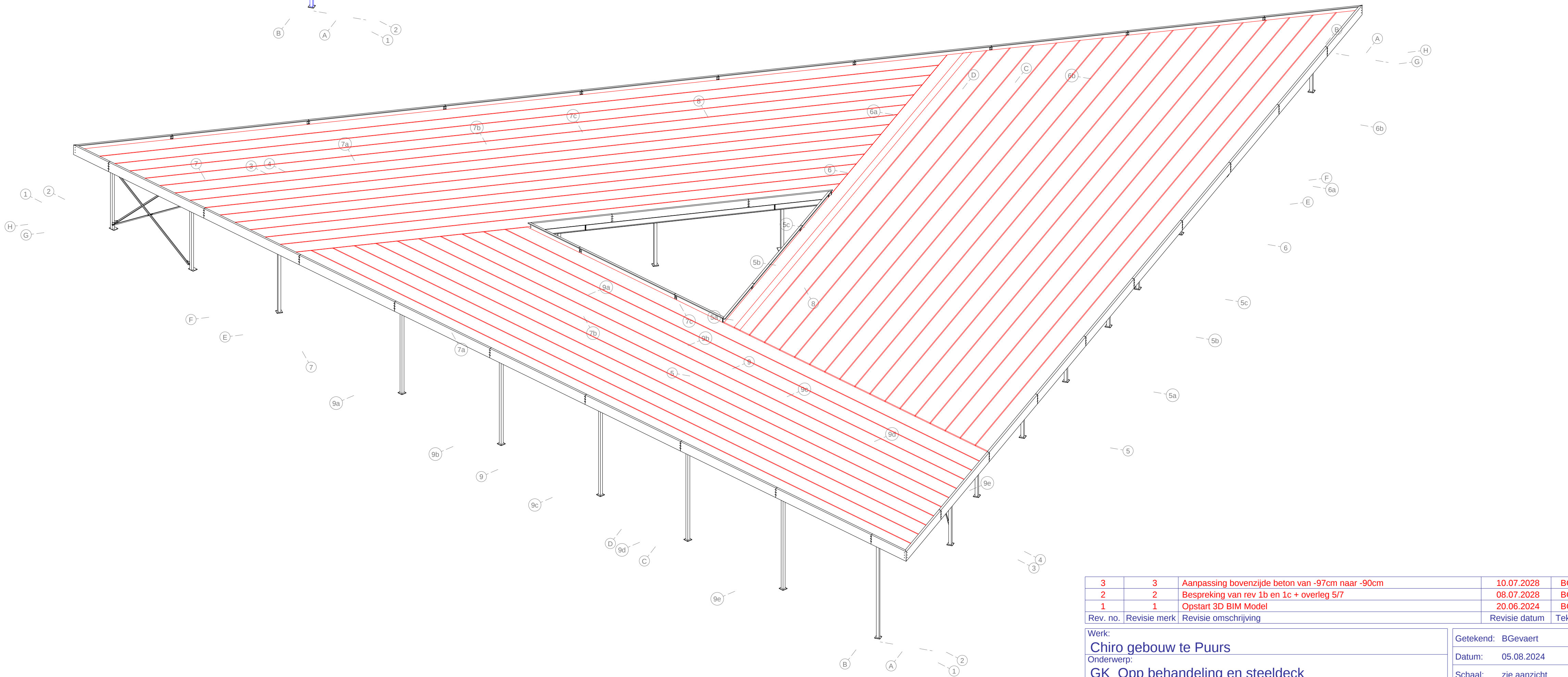
3D zicht - steeldeck draagrichting
