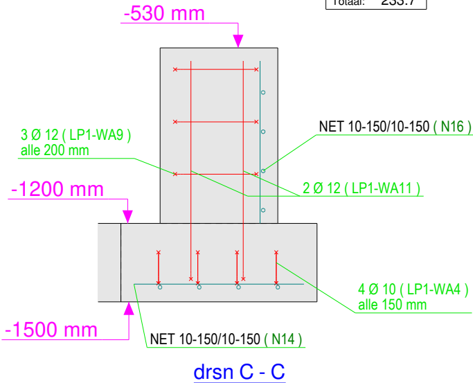
drsn C - C
