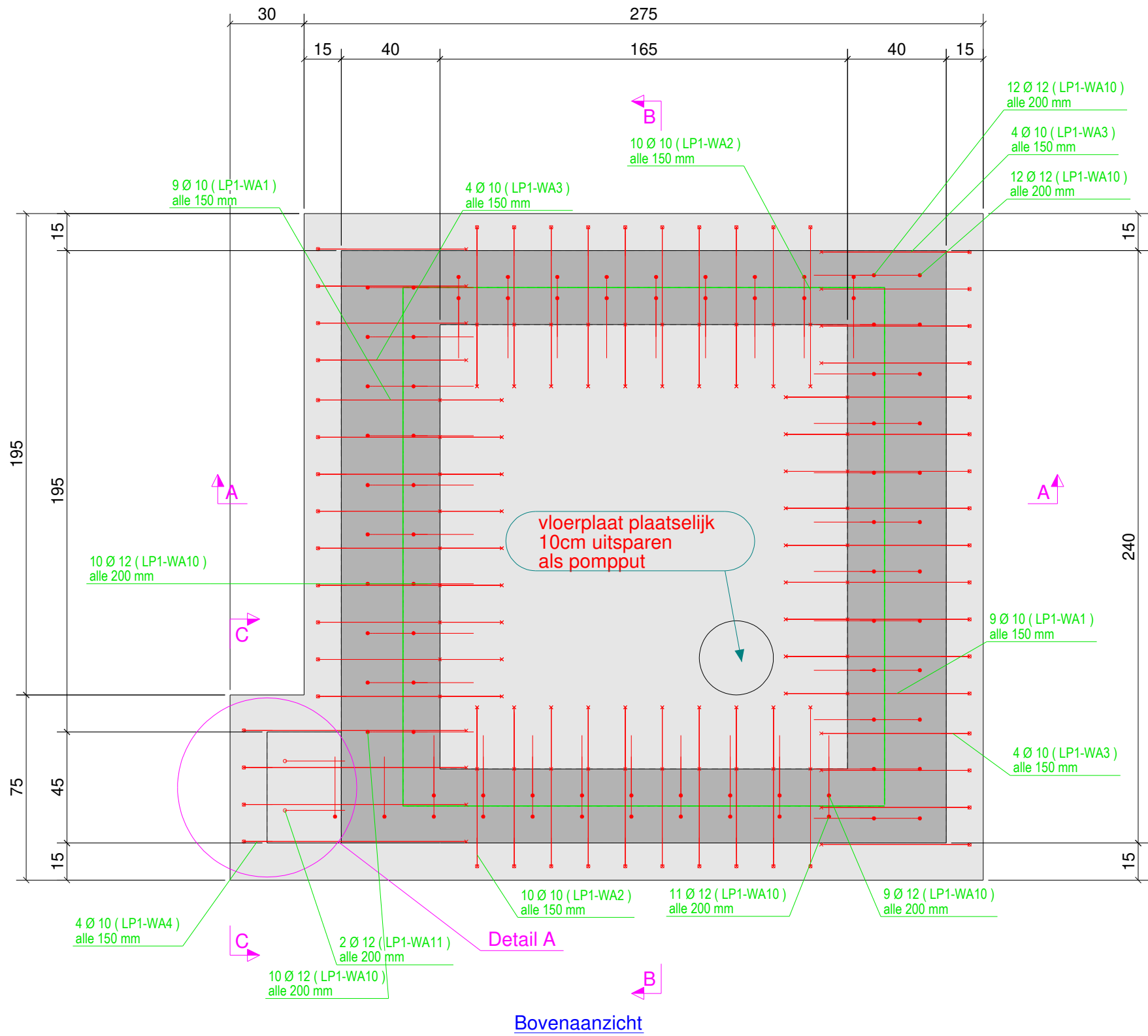
Bovenaanzicht
