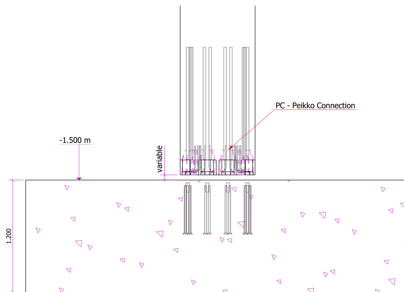
DETAIL A-A 1:25
