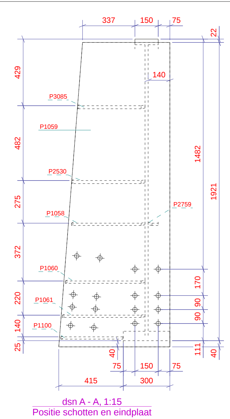
dsn A - A, 1:15 Positie schotten en eindplaat
