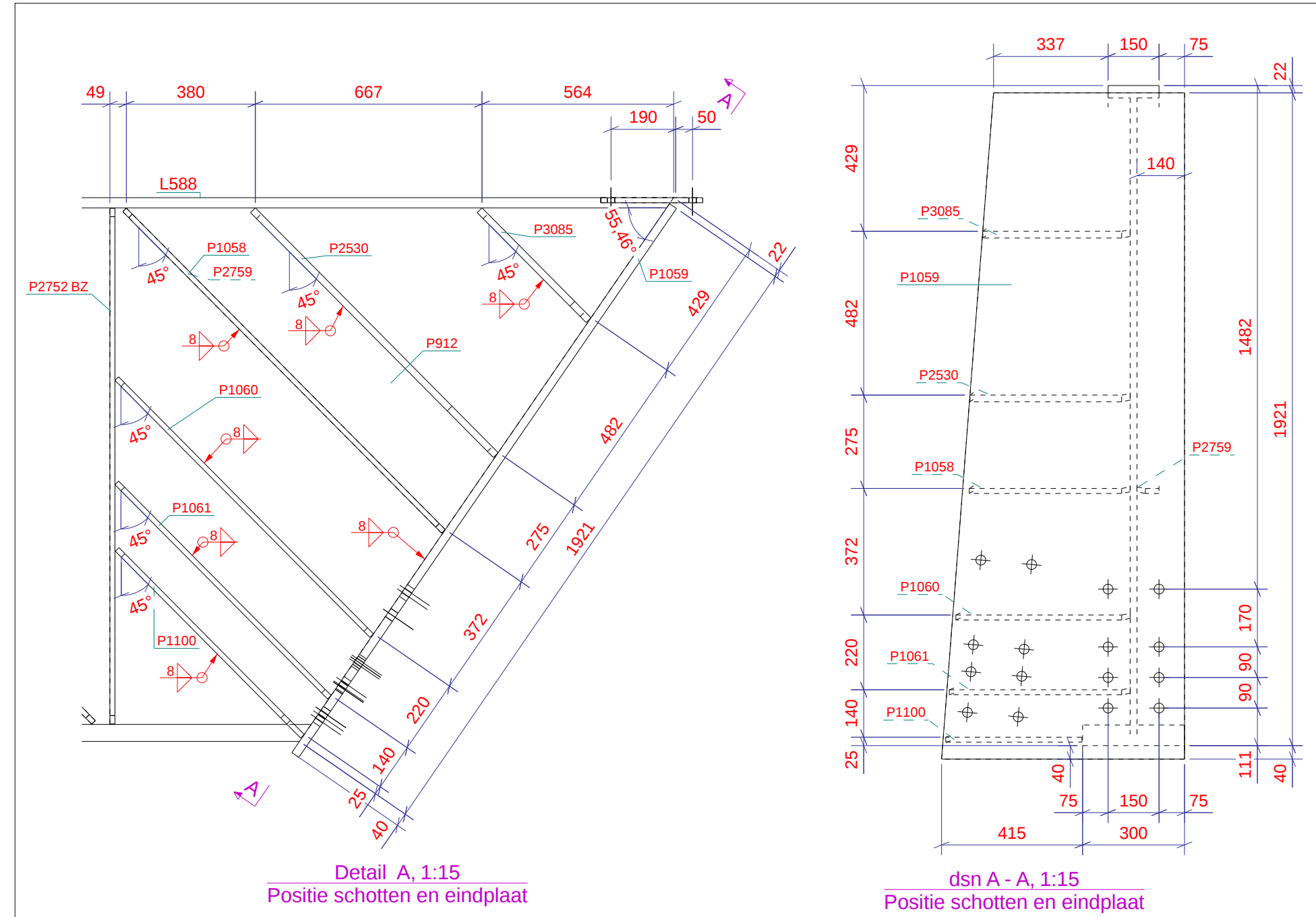
Detail A - A, 1:15 Positie schotten en eindplaat
