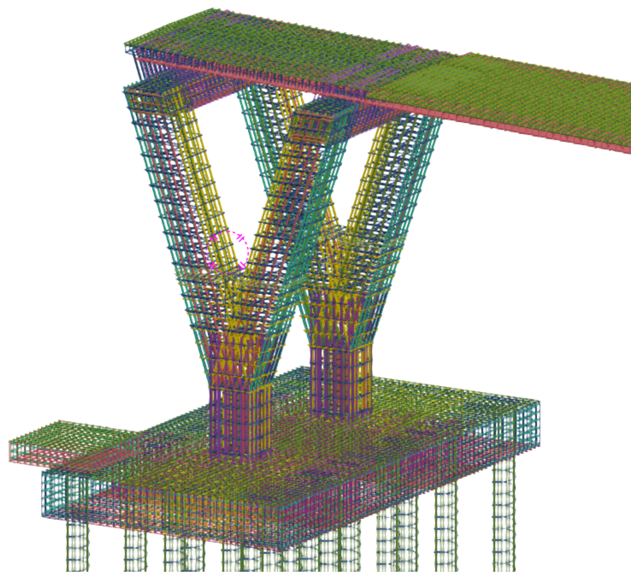
NOORD PERSPECTIEF OOSTZIJDE V-pijler (waping)
