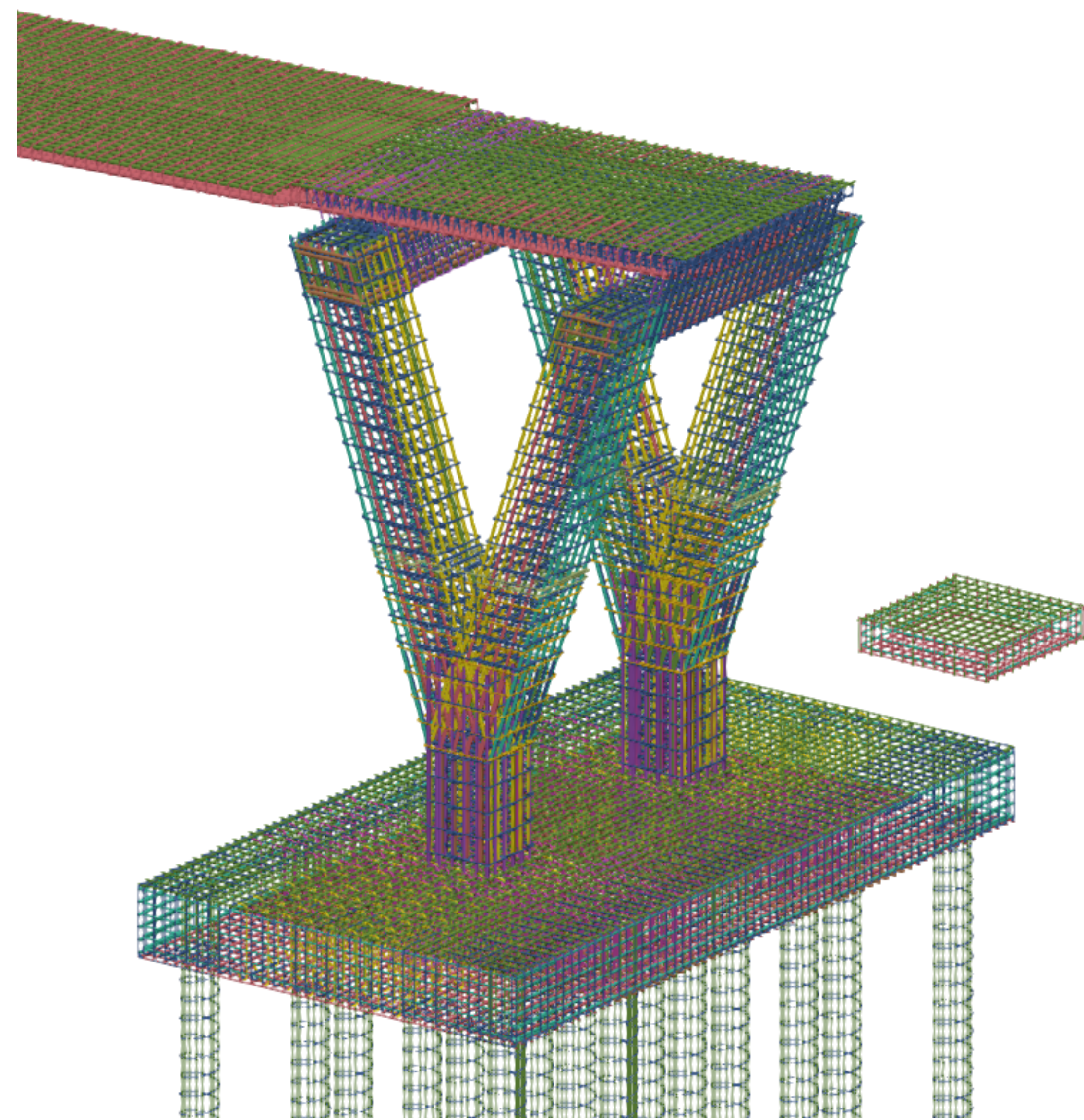
NOORD PERSPECTIEF WESTZIJDE V-pijler (waping)
