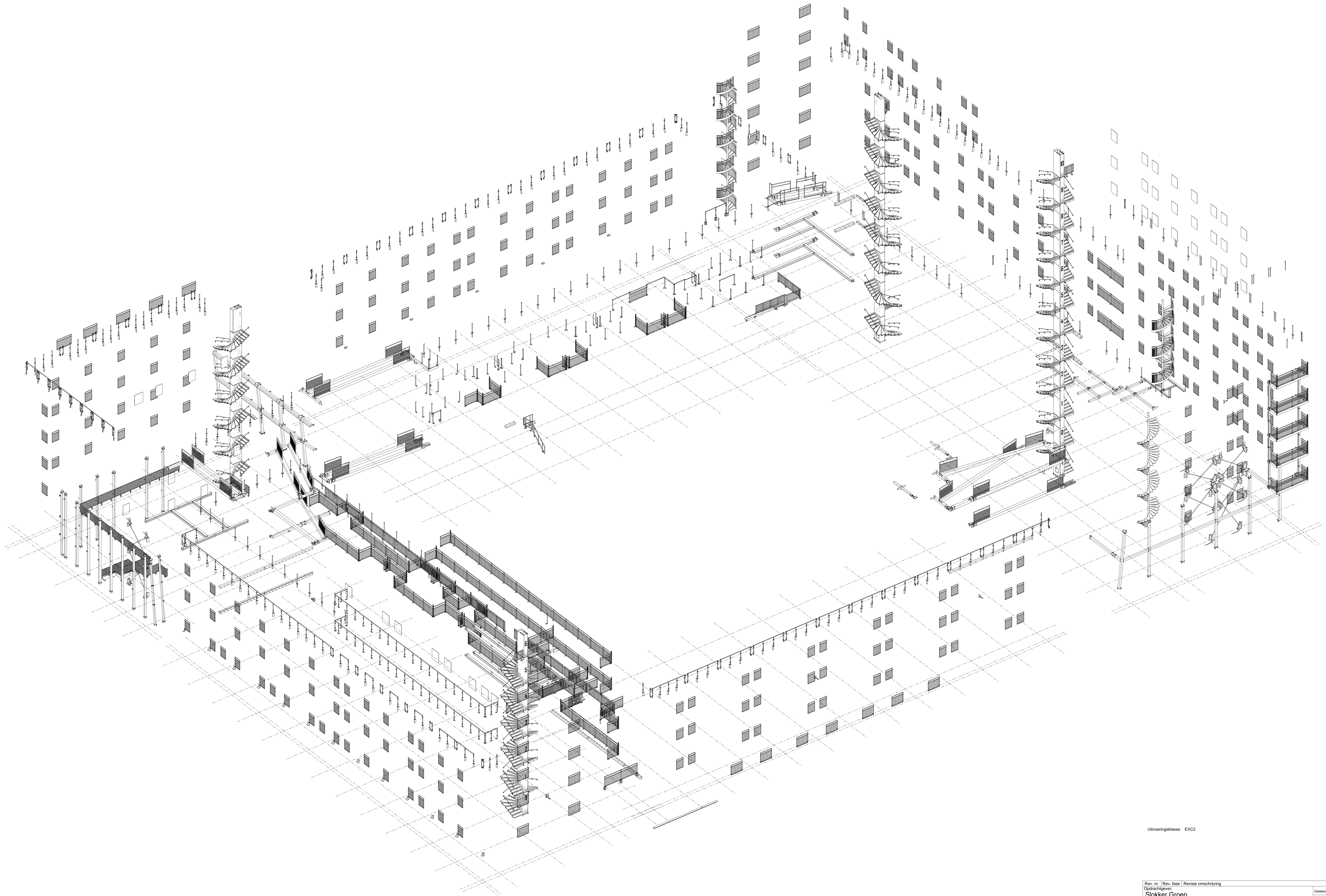
3D, 1:120
