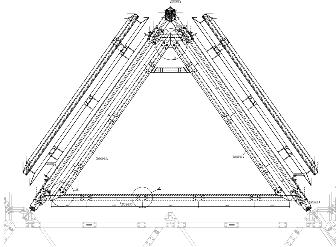
Ansicht auf Wand 1:10
