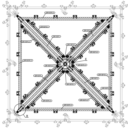
Draufsicht - Spitze Tropenhaus und Kakteenhaus 1:25
