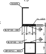
1-1 1:5
