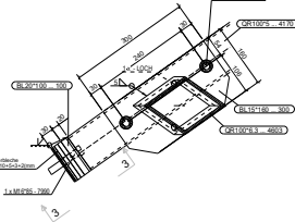
2-2 1:5
