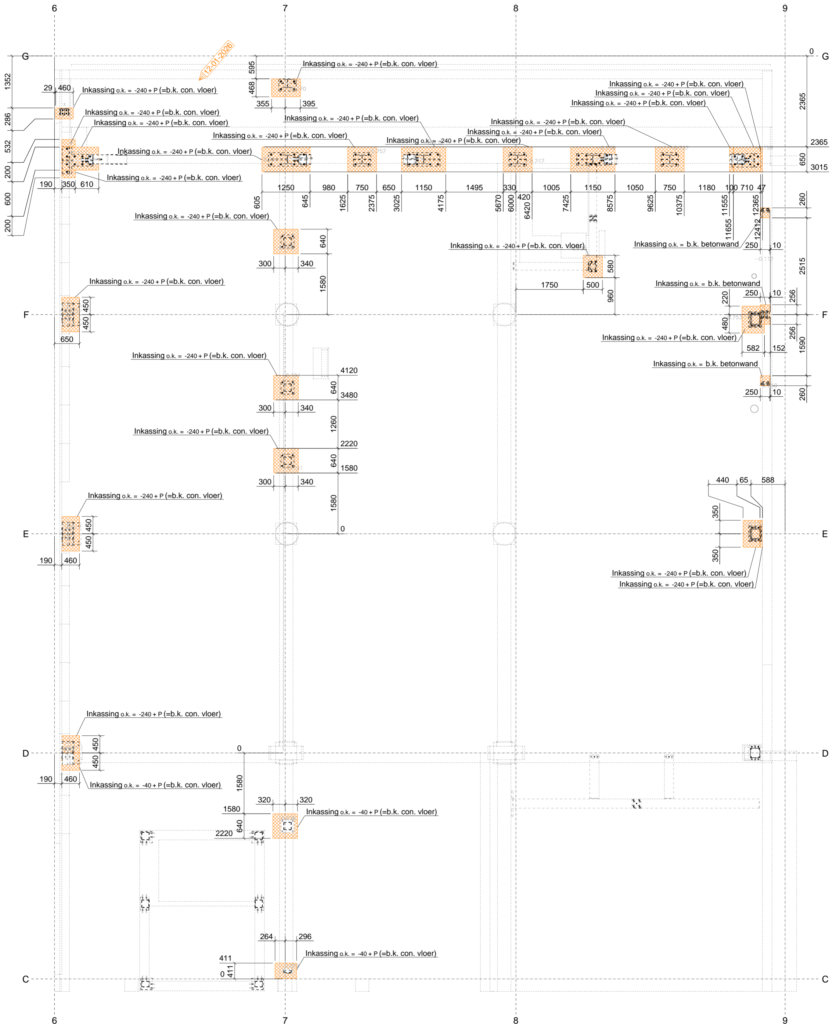
Sparingen en inkassingen -240, 1:60 Begane grond Renssenstraat
