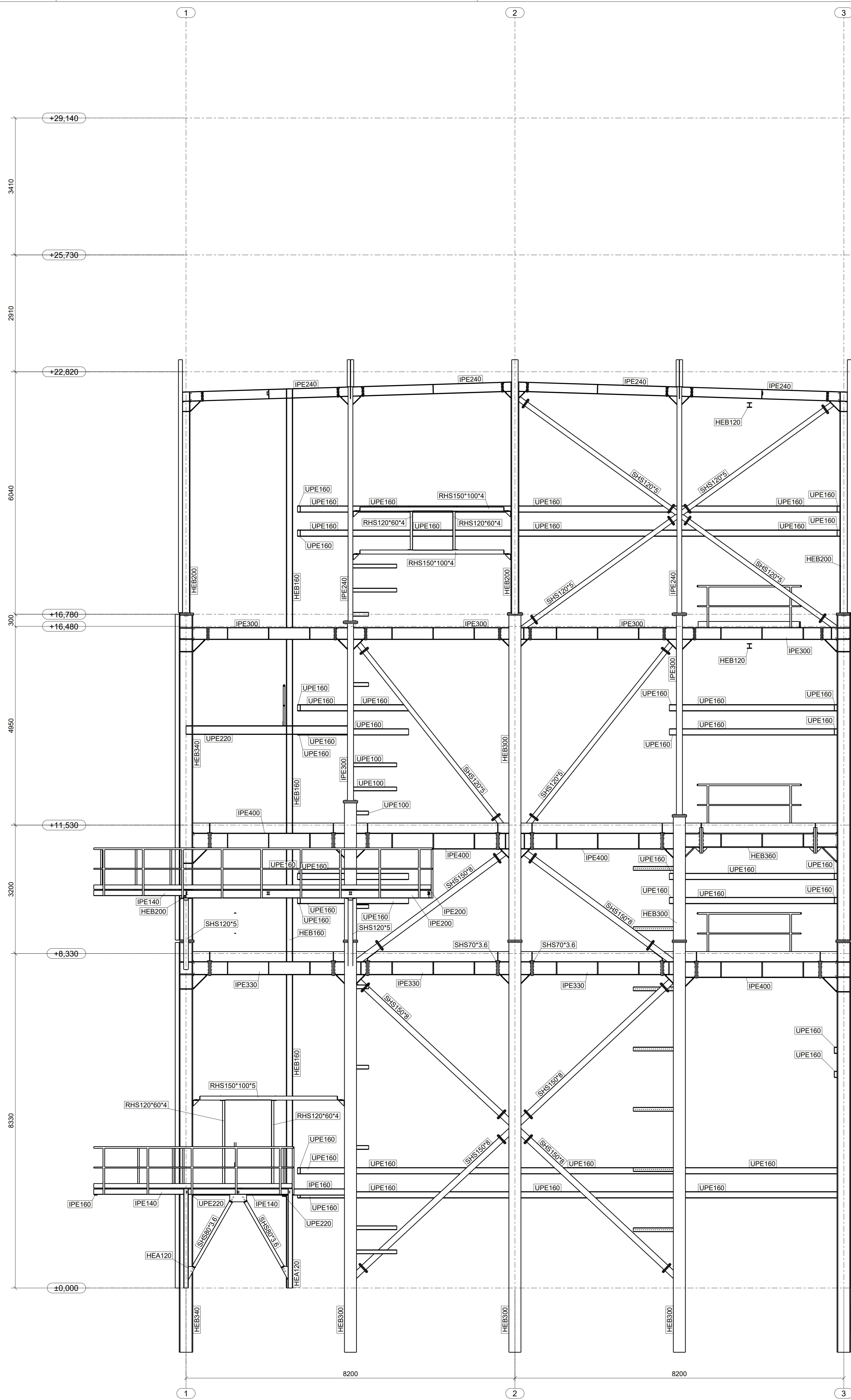
OSAA - VNĚJŠÍ POHLED 1:50
