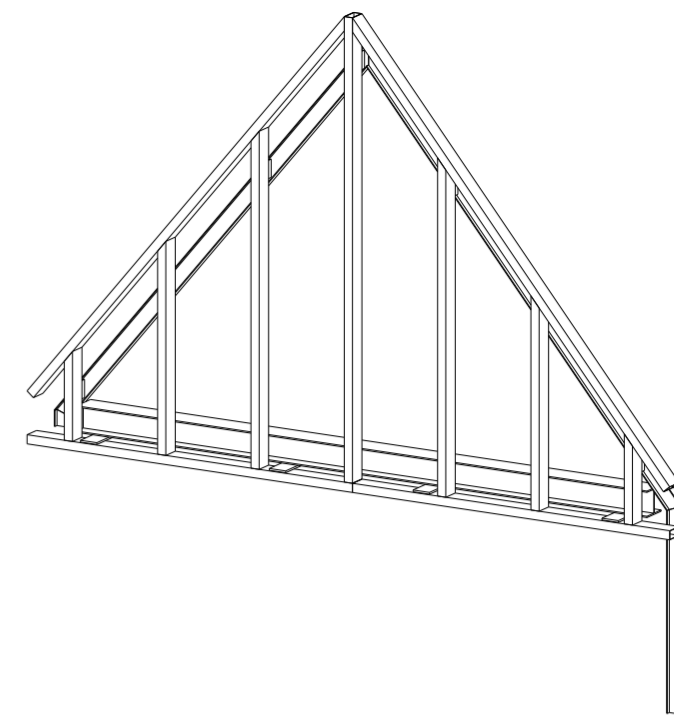
Bovenaanzicht 1:80
