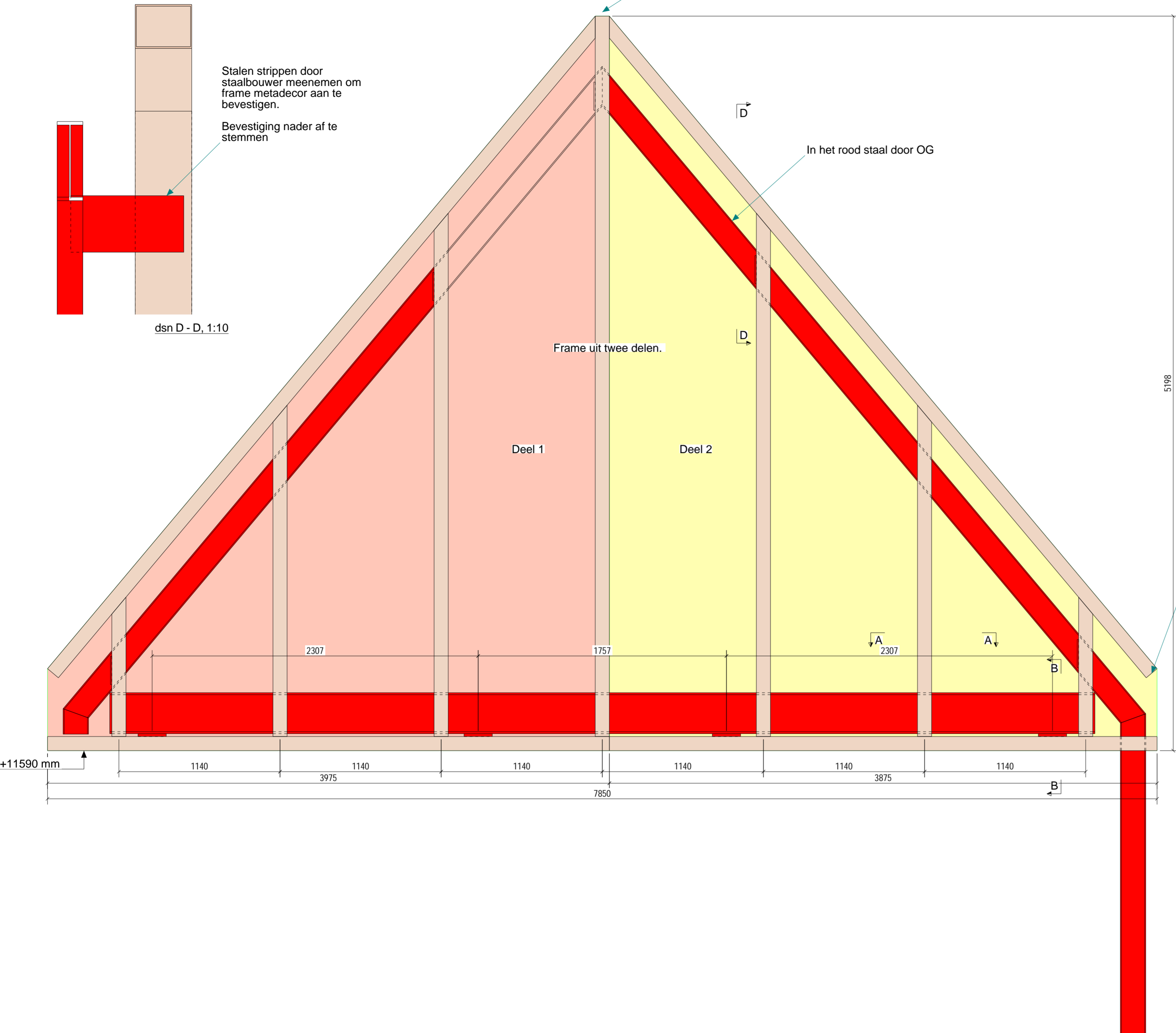
Vooranzicht - Daktheather Schaal 1:20
