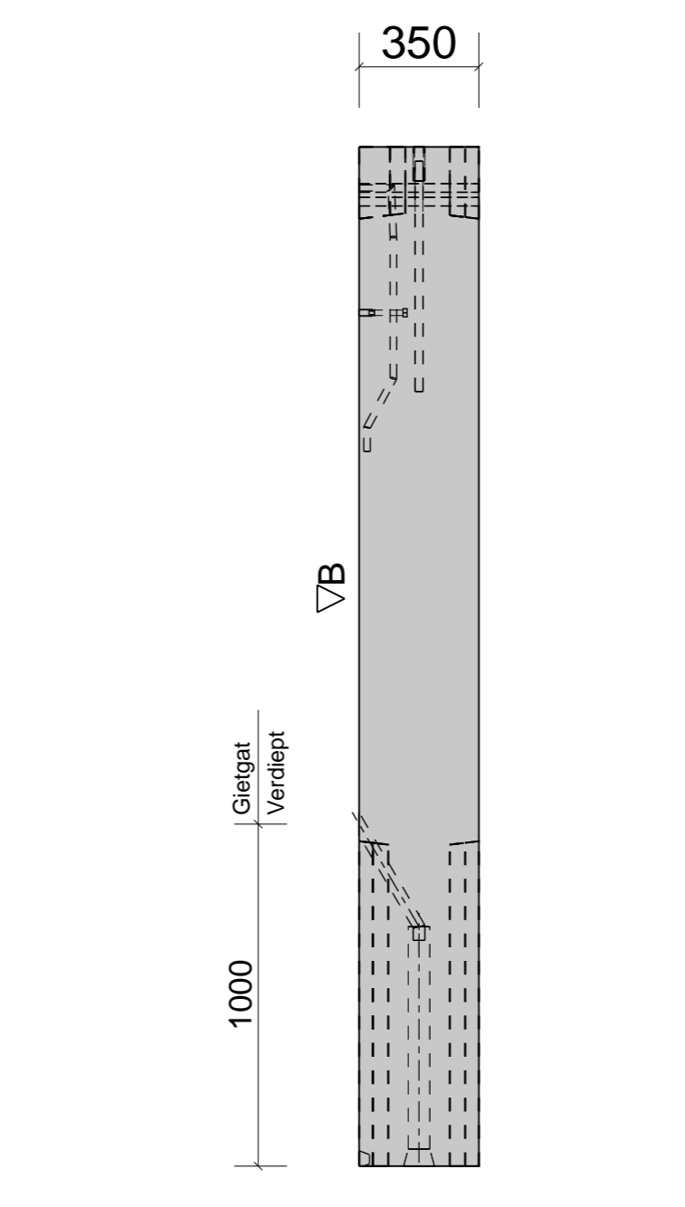
Doorsnede C LET OP: Ter verduidelijking, ankerplaten en elektro NIET zichtbaar
