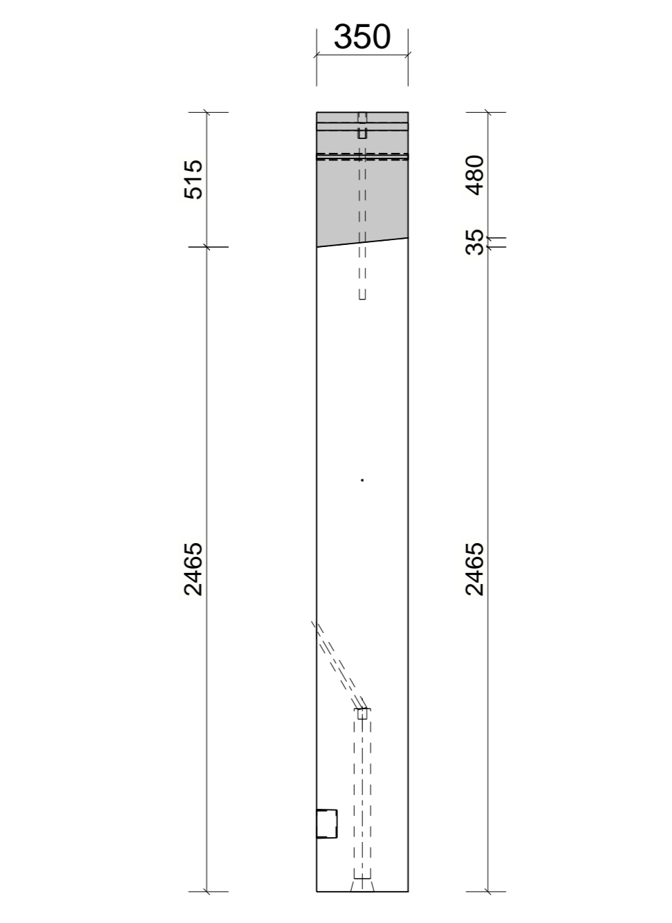
Doorsnede D LET OP: Ter verduidelijking, ankerplaten en elektro NIET zichtbaar
