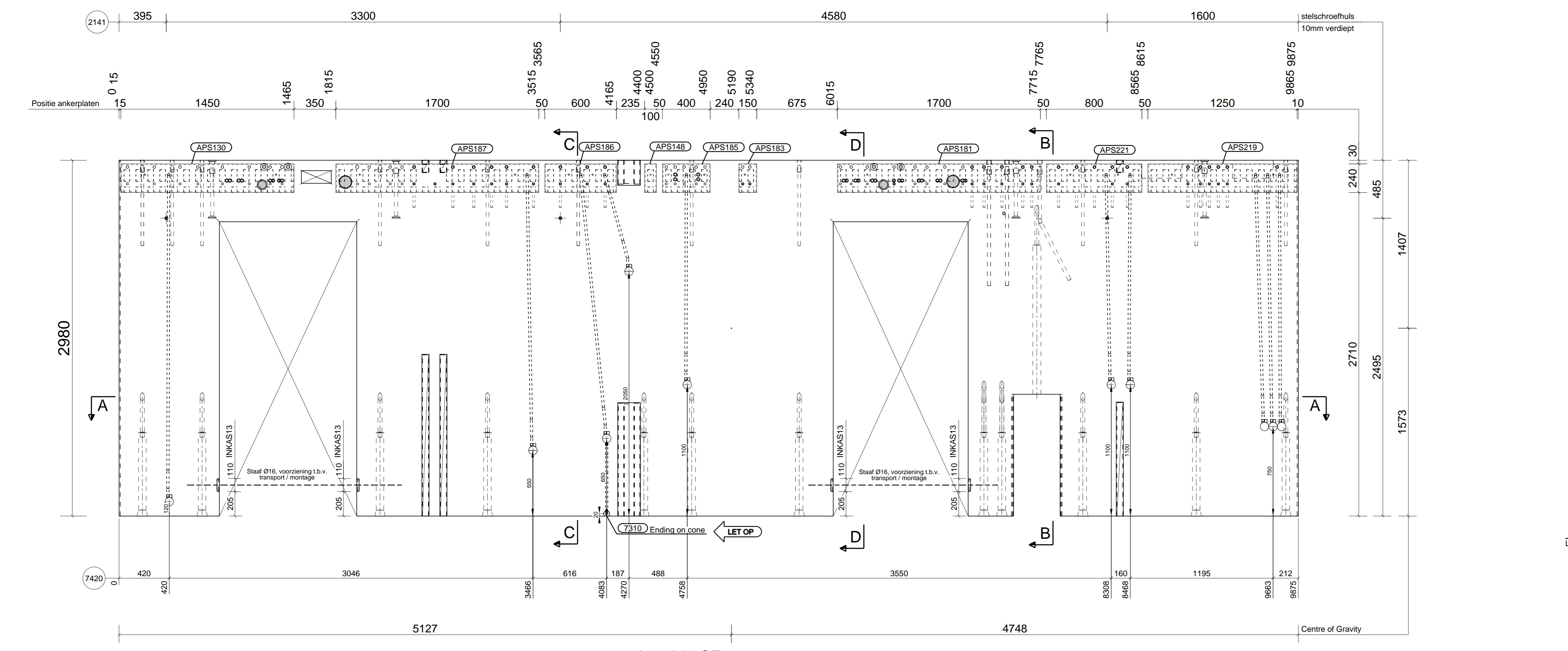
Aanzicht SZ (StortZide) LET OP: Zie bovenaanzicht, hoogte van StortZide (SZ SZ lijn) tot MB-MB lijn
