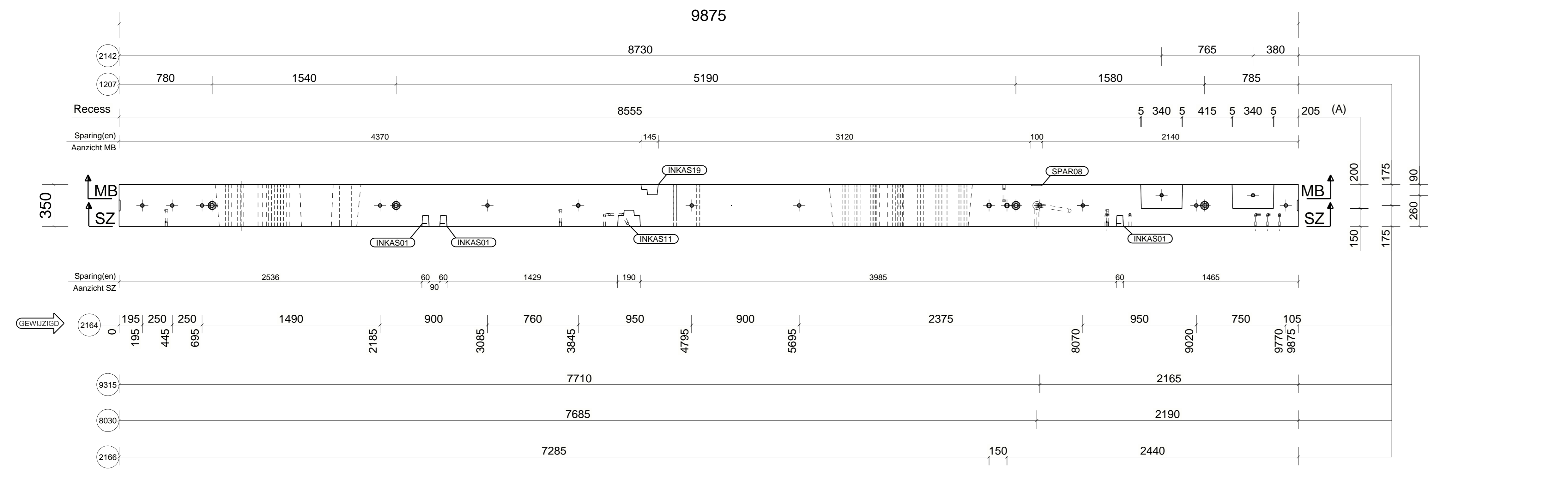
Bovenaanzicht LET OP: Ter verduidelijking, ankerplaten en elektro NIET zichtbaar
