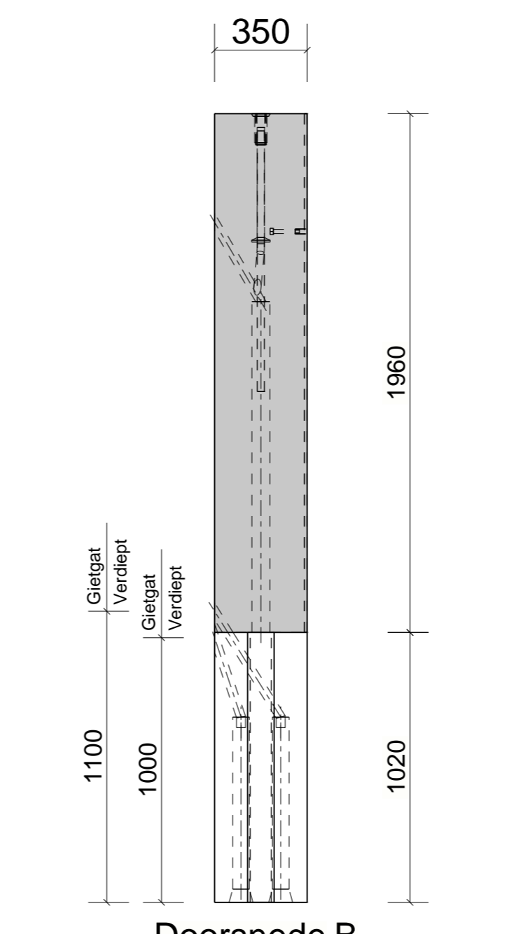
Doorsnede B LET OP: Ter verduidelijking, ankerplaten en elektro NIET zichtbaar
