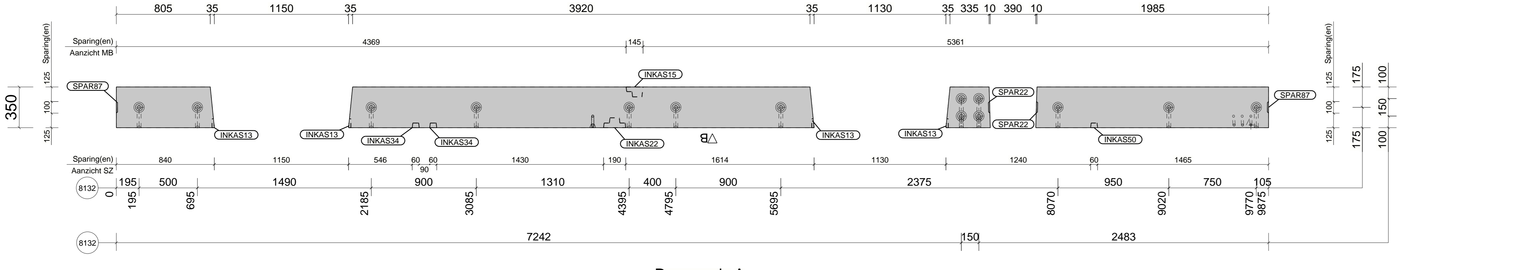
Doorsnede A LET OP: Ter verduidelijking, elektro NIET zichtbaar
